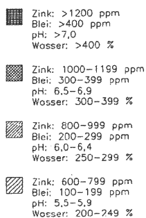
Abb. 2: Verbreitungsmuster der pflanzenverfügbaren Zink- und Bleigehalte, von pH-Wert und aktuellem Wassergehalt im Boden von 5 m x 5 m-Plots im NSG „Waldwiese im Wäschelbachtal“.
