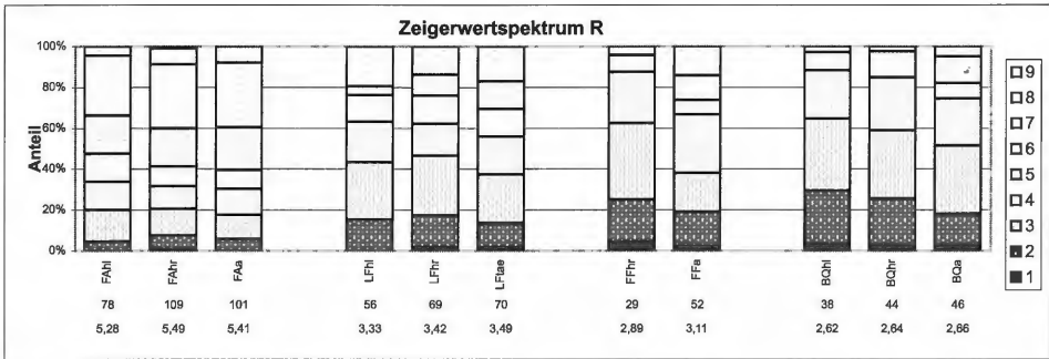
Abb. 14: Spektra der Reaktions-Zeigerwerte historischer (jeweils die beiden linken Säulen eines Blocks) und aktueller Aufnahmen (rechte Säulen(n) der Blöcke) des Galio odorati-Fagion (FA) Luzulo-Fagetum (LF), der Fichtenforste (FF) und des Birken-Eichen-Waldes (BQ) des Untersuchungsgebietes.
