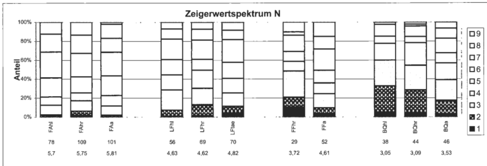
Abb. 16: Spektren der Stickstoff-Zeigerwerte historischer (jeweils die beiden linken Säulen eines Blocks) und aktueller Aufnahmen (rechte Säulen(n) der Blöcke) des Galio odorati -Fagion (FA) Luzulo -Fagetum (LF), der Fichtenforste (FF) und des Birken-Eichen-Waldes (BQ) des Untersuchungsgebietes.
