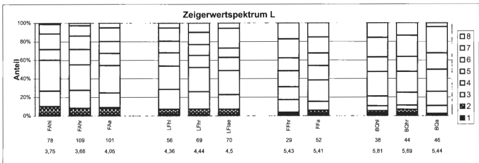
Abb. 11: Spektren der Licht-Zeigerwerte historischer (jeweils die beiden linken Säulen eines Blocks) und aktueller Aufnahmen (rechte Säulen(n) der Blöcke) des Galio odorati-Fagenion (FA) Luzulo-Fagetum (LF), der Fichtenforste (FF) und des Birken-Eichen-Waldes (BQ) des Untersuchungsgebietes.
