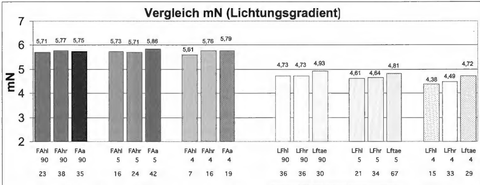
Abb. 21: Abhängigkeit des mittleren Stickstoffzeigerwertes historischer (jeweils die beiden linken Säulen eines Blocks) und aktueller Aufnahmen (rechte Säule der Blöcke) des Galio odorati-Fagenion (FA) und Luzulo-Fagetum (LF) in Abhängigkeit vom Lichtungsgradienten. Die Zahlen unter den Säulen geben die Deckungsgradklassen (K90 \geq 90%, K5 \geq 75%, K4 < 75% Deckung BS) sowie die Anzahl der Aufnahmen an.
