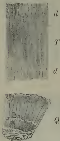
Calamites cf. lineatus Cotta sp. Im Museum der k. k. geolog. Reichsanstalt von Neu-Paka. — Q Querschnitt; T tangentiale Schlifffläche mit 2 Internodiallinien d und T . Die vertikalen Striche in T bedeuten die Primär-Markstrahlen; deren untere Enden je eine kleine Erweiterung bemerken lassen, die den Blattknospen entspricht; die oberen Enden der Primär-Markstrahlen sind aber auch mit einer kaum merkbaren Erweiterung versehen, die die Wurzelknospe bedeutet.
