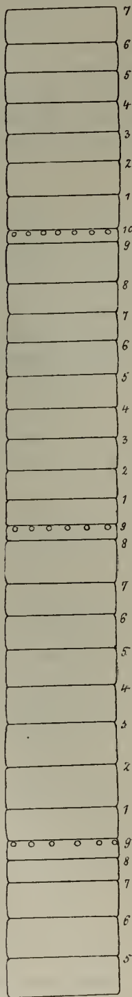
Calamites Schützei Stur. Der von Goeppert erworbene im Breslauer Mineralogischen Mu- seum ausgetellte Stamm. 1mm = 1cm der Natur.
