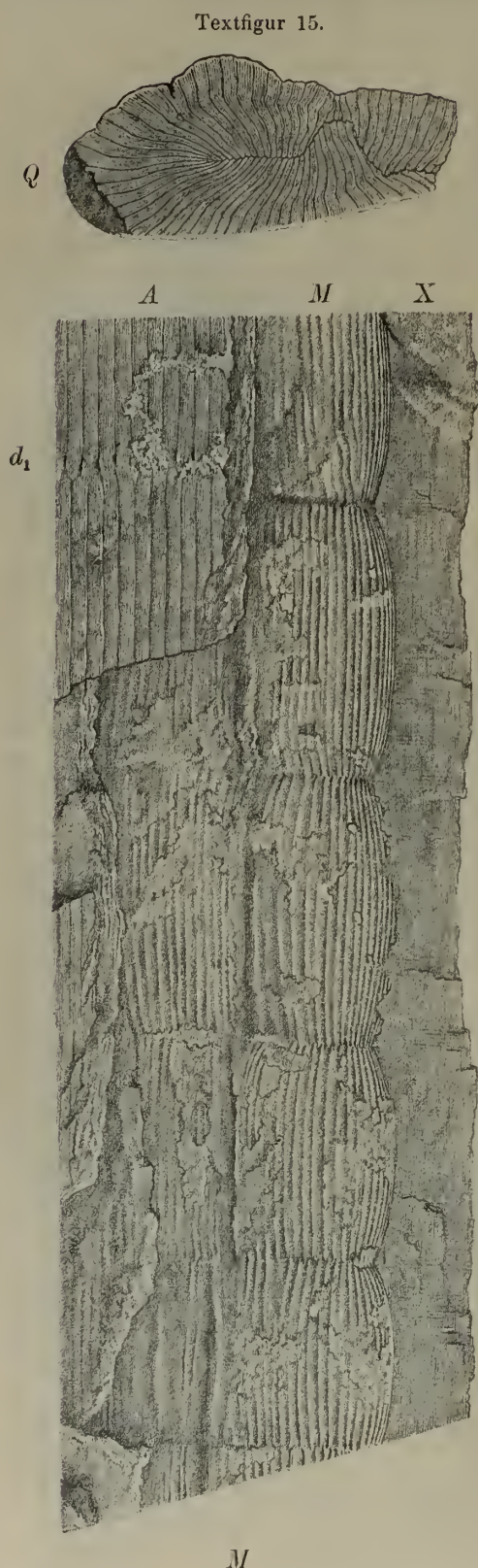
Calamites sp. aus der Verwandtschaft des Calamites Suckowii Bgt. — Neu-Paka in Böhmen, gesammelt von Jos. Jampilek. — A äussere Oberfläche des Holzkörpers; M die Wand der Markhöhle; X die Dicke des Xylems; d d die Internodallinien der Markhöhlenwand; d 1 eine Internodallinie der äusseren Oberfläche A mit erhaltener Blattknospenreihe.
