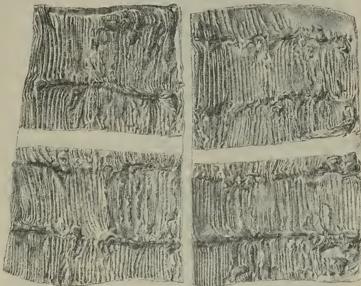
Calamites bistriatus Cotta sp. Dasselbe Stück wie Textfigur 6. Aufgewickelter Abguss der Centralhöhle. Man sieht, dass die Internodiallinien kräftige Einschnürungen des Steinkernes hervorrufen. Rechts von der Mediane der Figur ist die Rippung der Centralhöhle besonders gut erhalten, da hier der Abguss bei der Herausnahme ganz unverletzt blieb. Links im oberen Theile der Figur ist eine Astnarbe (Astursprung) mit der Convergenz zahlreicher Rippen sehr wohl abgedruckt.
