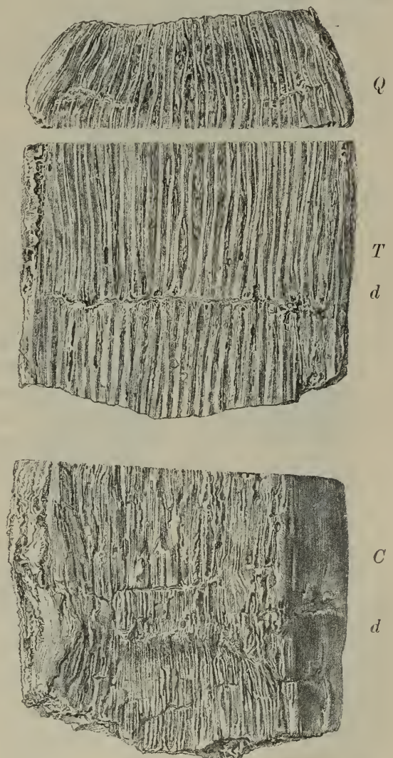
Calamites cf. bistriatus Cotta sp. Aus dem städtischen Museum in Chemnitz; von Chemnitz in Sachsen. — C Ansicht der Wand der Centralhöhle des Stückes mit bei d stark vorspringender Internodallinie. — T tangentielle Schlifffläche an der äusseren Umgrenzung des Stückes. — Q Querschnitt des Stückes.
