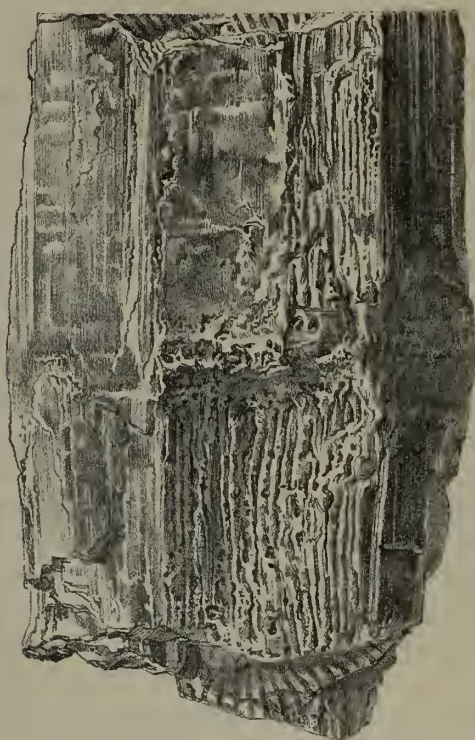
Calamites striatus Cotta sp. Aus dem städtischen Museum in Chemnitz; von Chemnitz in Sachsen. — C Ansicht der gerippten Wand der Centralhöhle und der rechts und links davon liegenden Radial-Spaltflächen. Bei d eine Internodallinie, die vielfach ausgebrochen ist; darunter ist die Wandfläche der Centralhöhle gerippt, während darüber nur rechts die Rippung wahrnehmbar ist, links dagegen ist sie von einer glatten Quarzfläche verdeckt. Oben und unten sieht man im Querschnitt die zweierlei Streifen, dunklere und lichtere in Wechsel-lagerung.
