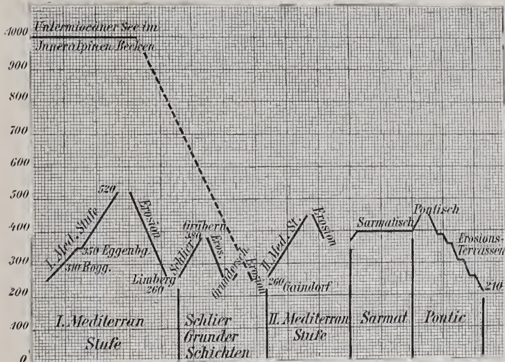
Diagramm der Wasserstandschwankungen im Wiener Becken zur Zeit des Miocäns und Pliocäns.
