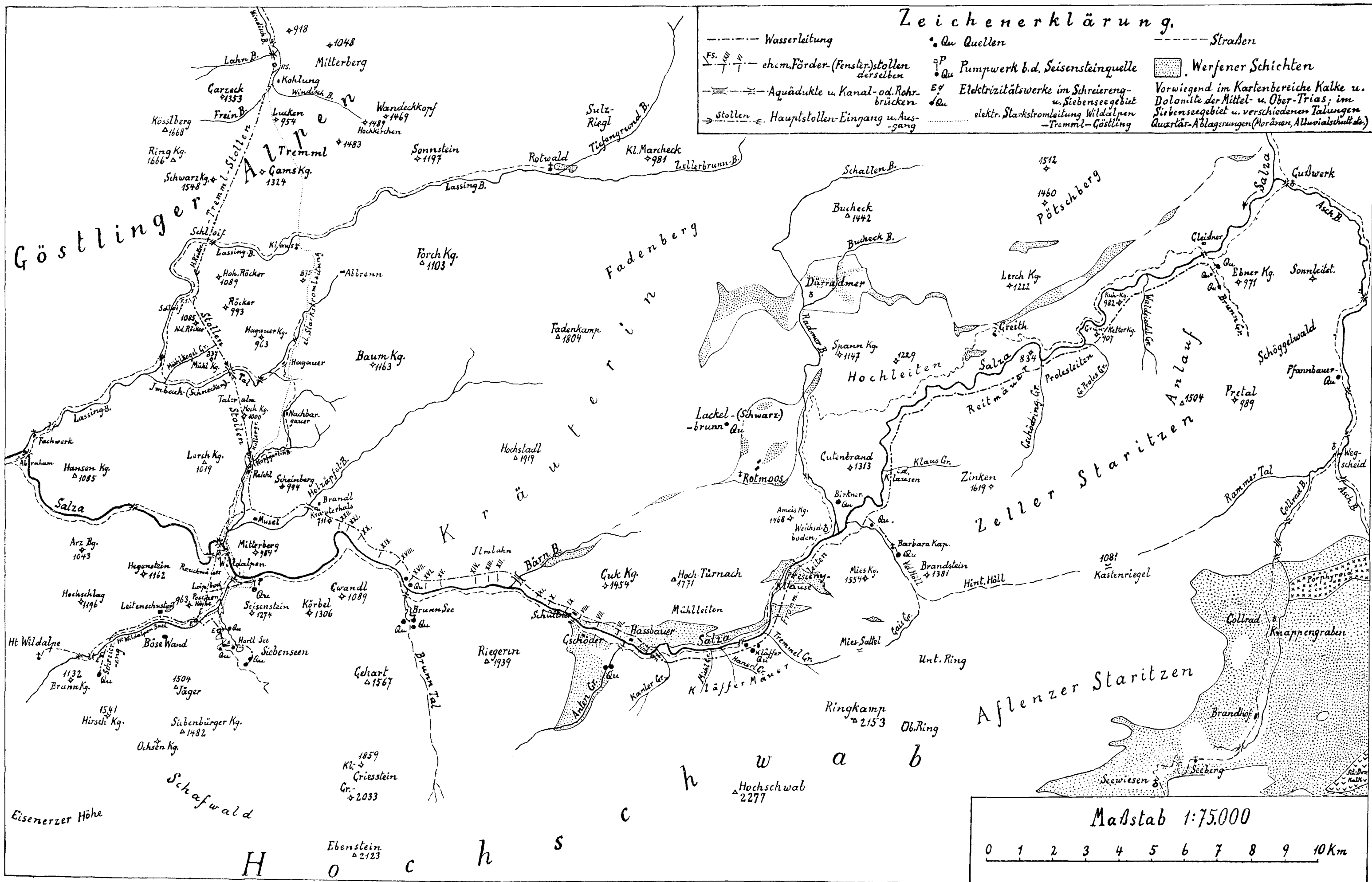
Verlauf der Zweiten Wiener Hochquellenleitung von den Quellen im Salzaal-Gebiet bis zum Windischbach N vom Tremmlstollen-Ausgang, entworfen von F. Trauth.
