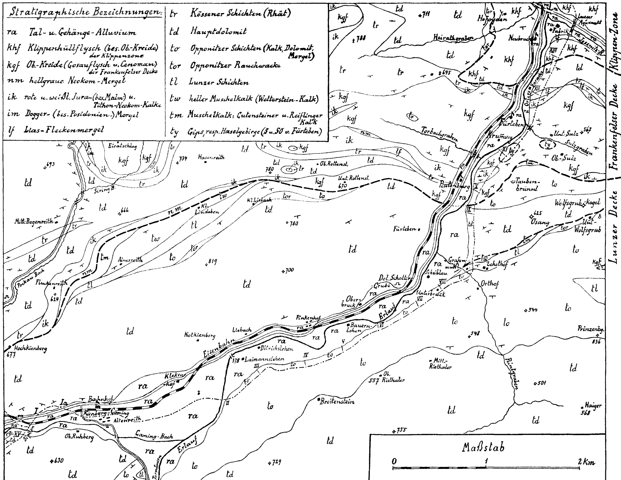
Geologische Karte des Erlaufthal-Gebietes zwischen Kienberg-Gaming und Neubruck mit der dortigen Wasserleitungsstrecke Aufgenommen von F. Trauth (Maßstab 1:25.000).
