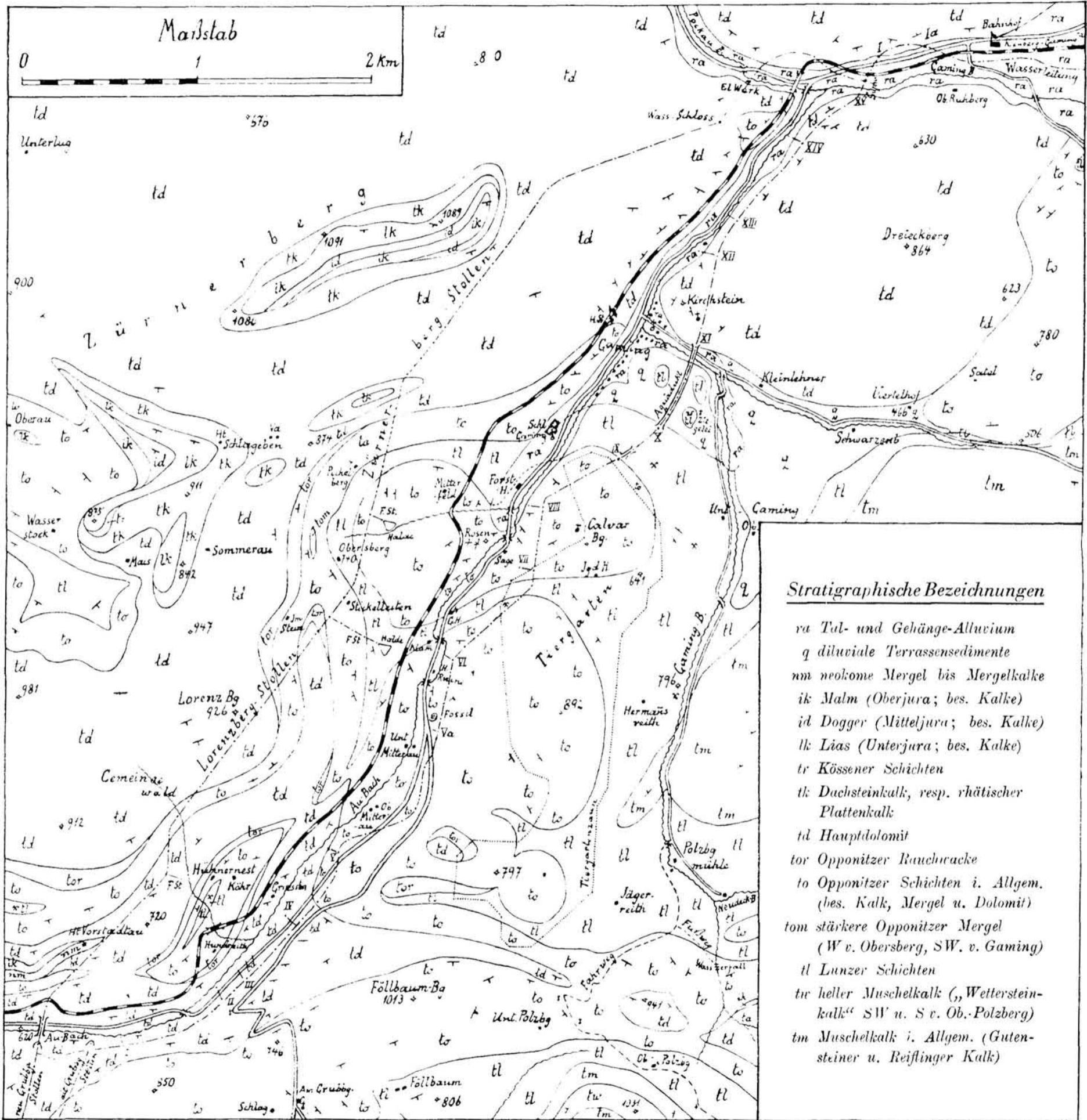
Geologische Karte des Au- (Mitterau-) und Gamingbach-Gebietes bei Gaming mit den dortigen beiden Wasserleitungsstrecken. Aufgenommen von F. Trauth (Maßstab 1:25.000).
