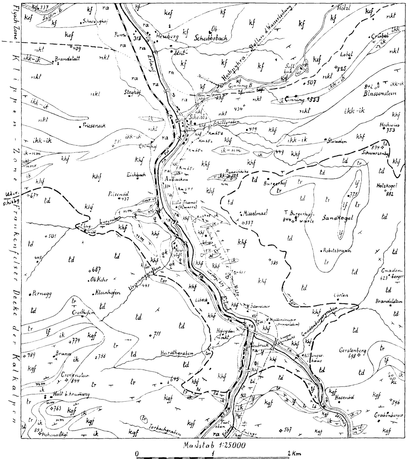
Geologische Karte des Erlaufal-Gebietes zwischen Fürteben bei Neubruck und Heuberg bei Scheibbs mit der dortigen Wasserleitungsstrecke. Bes. nach eigenen Aufnahmen und älteren F. Blaschke's entworfen von F. Trauth.
