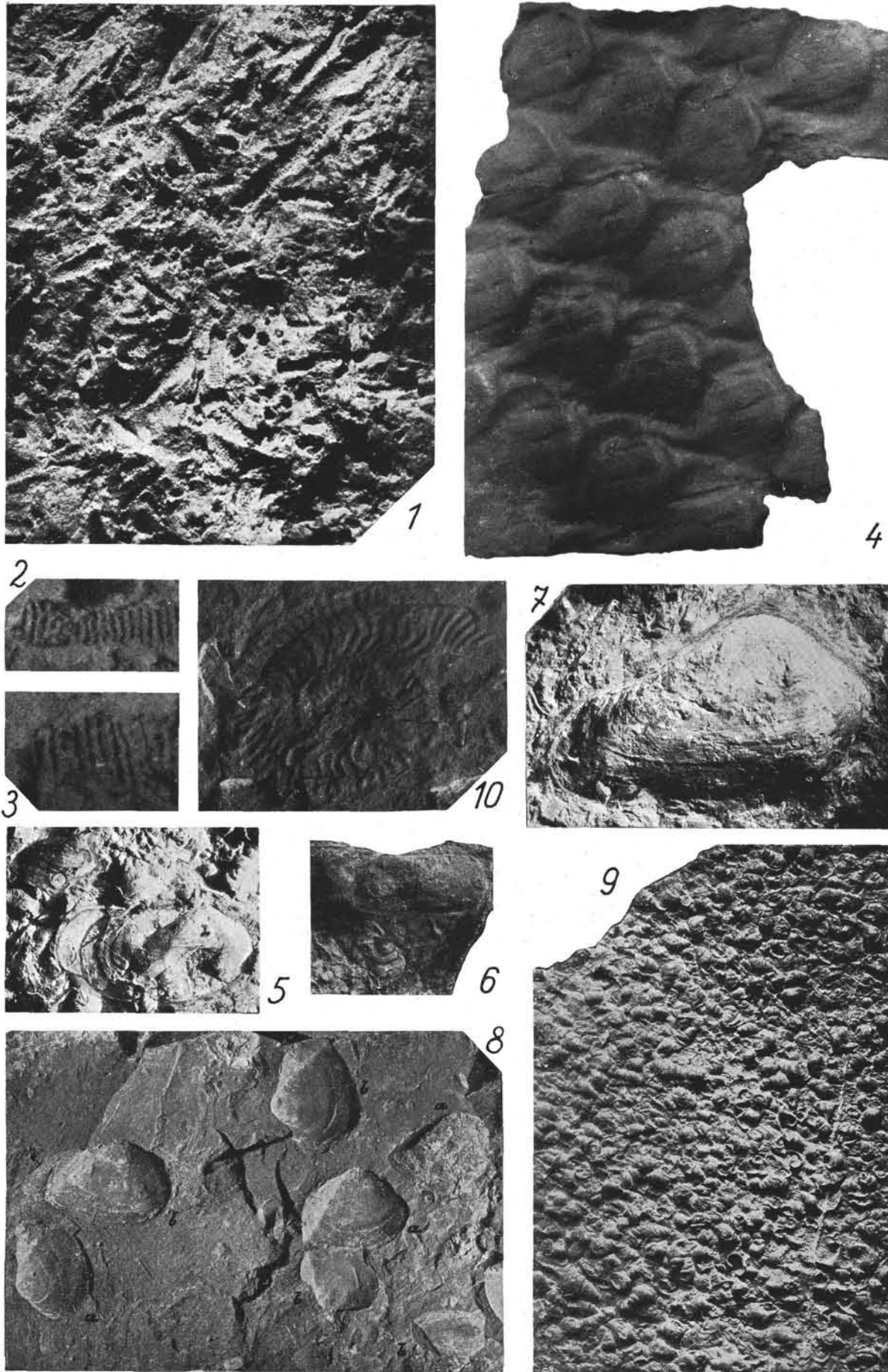
Fossilien aus der Trias- und Juraformation. (Fig. 1—4 zum Beitrag von E. Kamptner und E. Hofmann).
