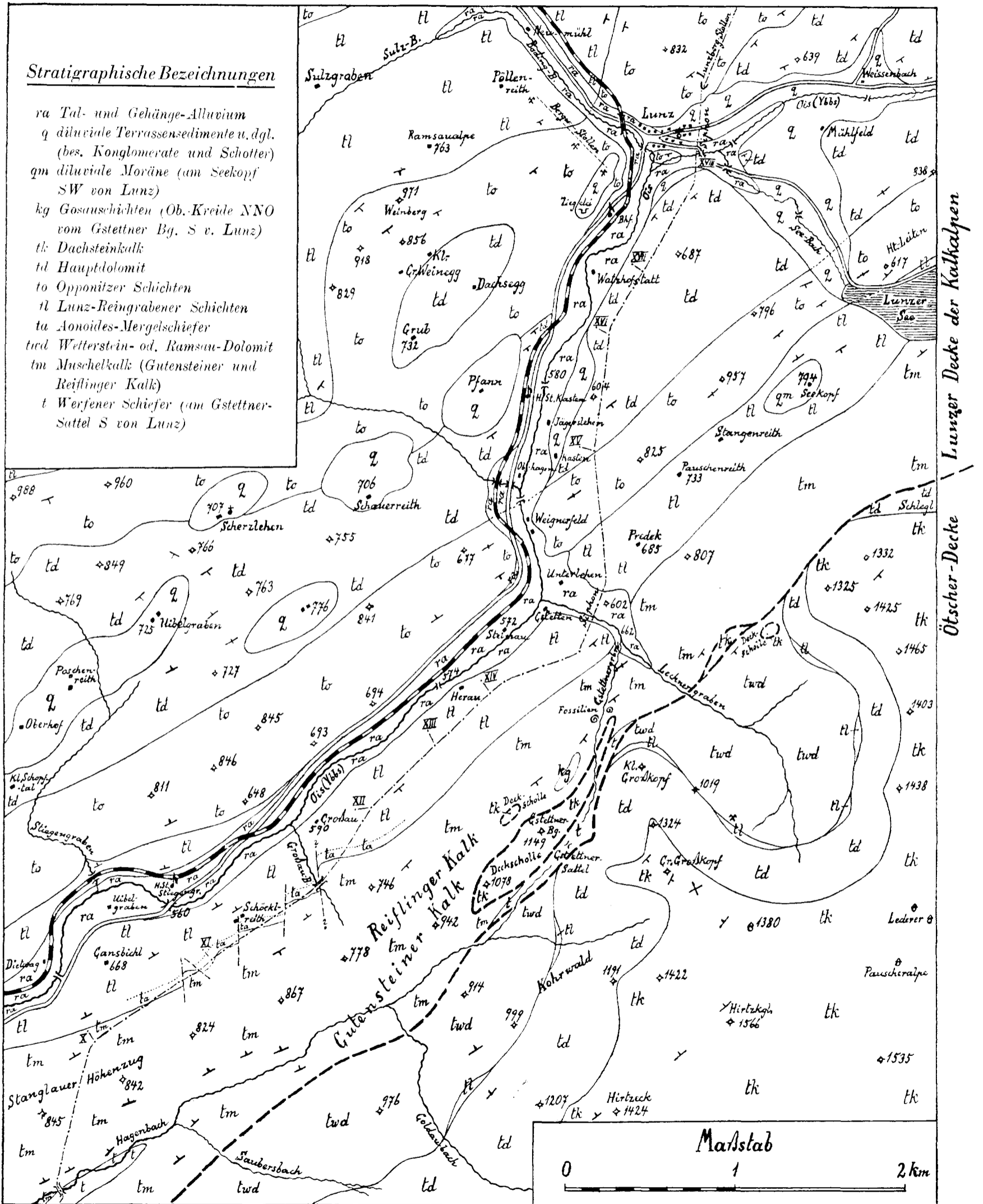
Geologische Karte des Ybbstal-Gebietes SW und S von Lunz mit der Wasserleitungsstrecke vom Hagenbach bis zum Lunzberg-Stollen. Aufgenommen von F. Trauth. (Maßstab 1:25.000).
