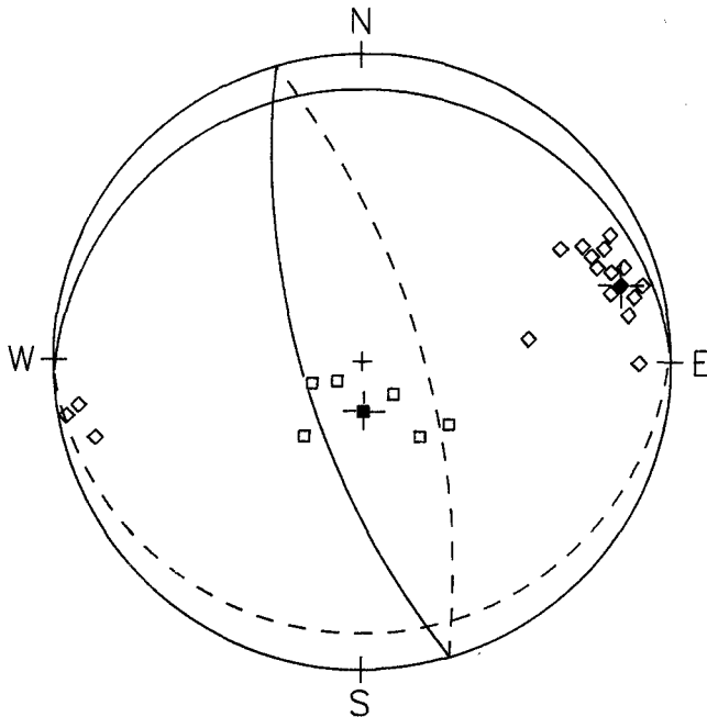
Abb. 7. Klufrächendiagramm in flächentreuer Projektion. ◇ = Pole der Klüftung k_a (untere Hälfte der Lagenkugel); □ = Pole der Klüftung k_b (untere Hälfte der Lagenkugel), ◆ = durchschnittlicher Pol von k_a ; ■ = durchschnittlicher Pol von k_b . Dargestellt sind auch die Großkreise der durchschnittlichen Richtungen von k_a und k_b .
