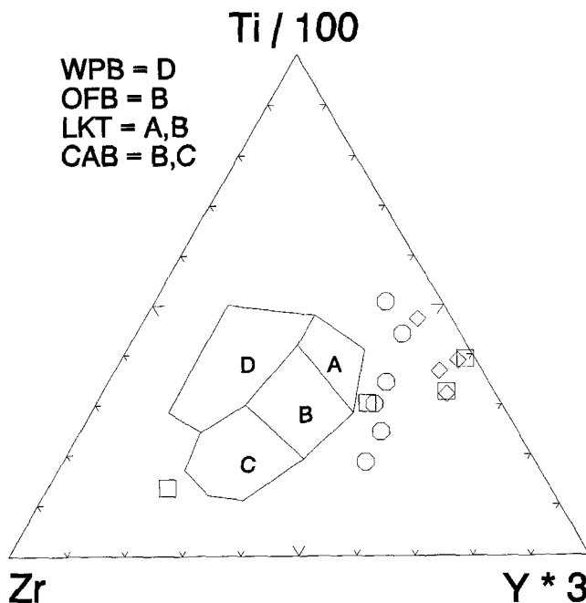
Abb. 11. Ti-Zr-Y-Dreieck nach PEARCE & CANN (1973). WPB = „Within-Plate“-Basalte; OFB = Ozeanbodenbasalte; CAB = Kalkalkali-Basalte; LKT = „Low-K“-Tholeiite.
