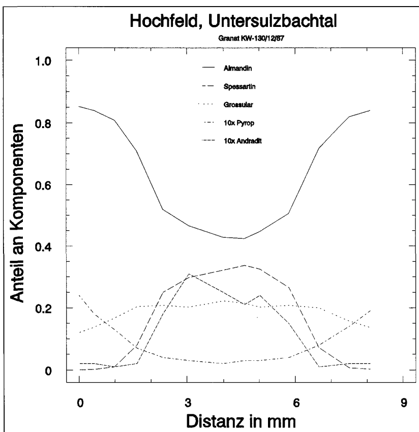
Abb. 8. Granatzonarbau in Quarzit. Probe KW 130-12/87. Pyrop- und Andraditkomponente 10-fach überhöht.
