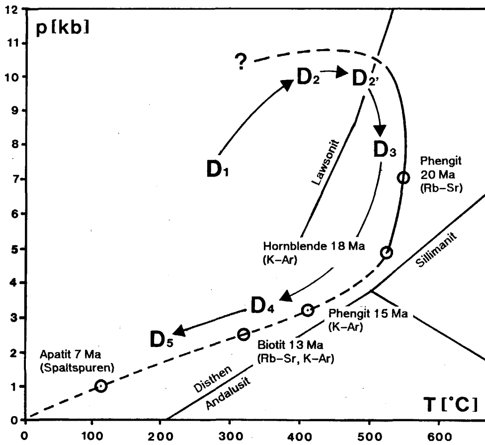
Abb. 6. PTtD-Pfad, basierend auf dem in LAMMERER & MORTEANI (1990) veröffentlichten, durch BLANKENBURG et al. (1989) modifizierten PTt-Pfad von SELVERSTONE et al. (1984).
