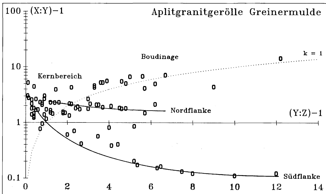
Abb. 4. Vergleichende Darstellung von 90 Strainanalysen an Aplitgranitgeröllen der D_2 -Greinermulde im logarithmischen Diagramm nach FLINN (1962).
