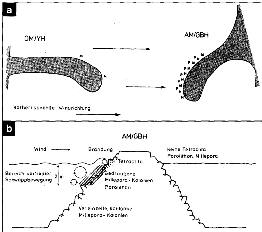
Abb. 1. Die Bedeutung hydrodynamischer Bedingungen für die Ansiedlung von riffbildenden Arten an künstlichen Riffmodellen bei Eilat (Rotes Meer).
