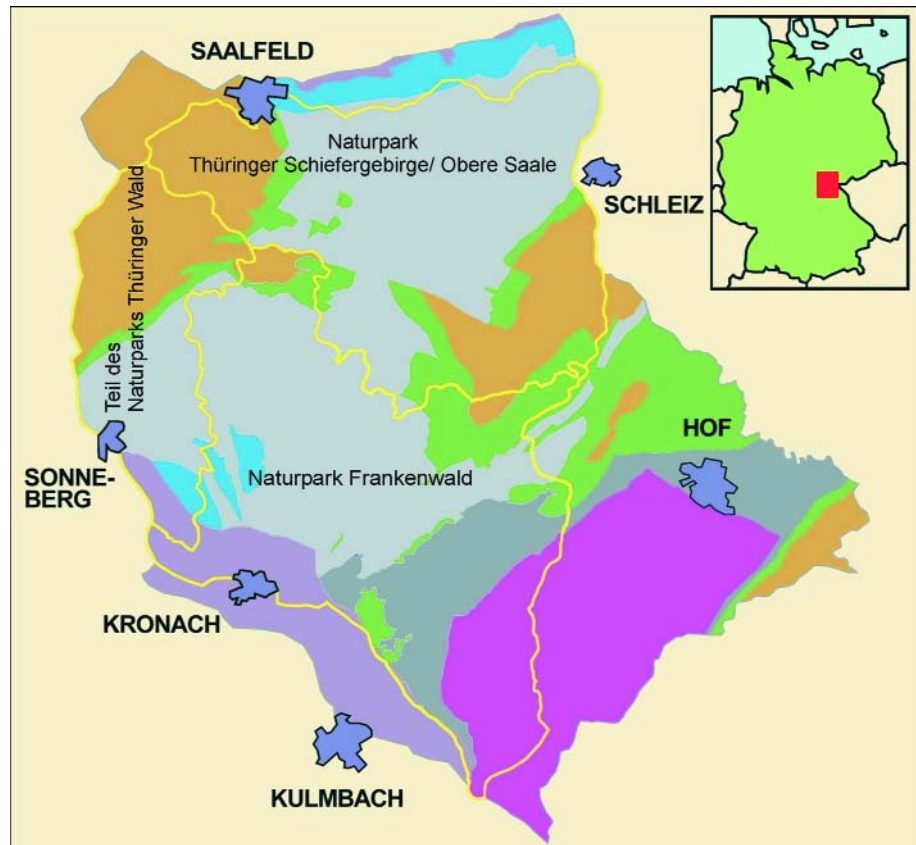
Abb. 1. Geologische Übersichtsskizze des geplanten Geopark-Gebietes. Das Kerngebiet der drei Naturparke ist gelb umrahmt. Braun: Ordovizium; grün: Devon; hellgrau: Karbon der „Thüringischen Fazies“; dunkelgrau: „Bayerische Fazies“ (Kambrium–Karbon); blau: Perm; rosa: Münchberger Gneismasse; violett: Trias.
