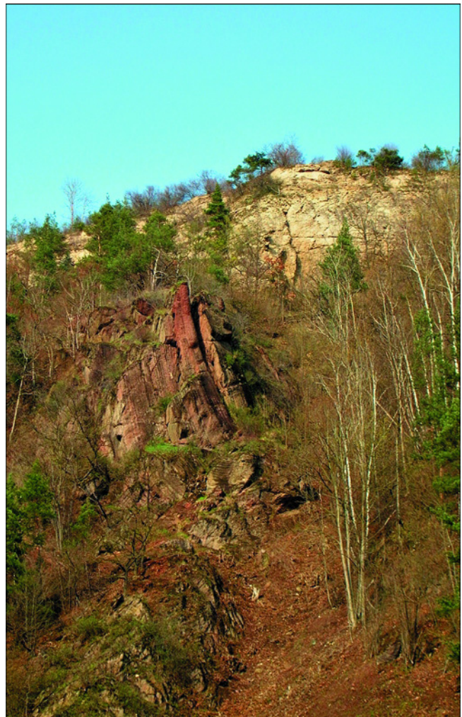
Abb. 2. Der Bohl bei Saalfeld ist wegen der Diskordanz von Zechstein-Kalkstein über gefaltetem variszischem Grundgebirge weltbekannt und gehört zu den 77 bedeutendsten Geotopen Deutschlands. Bildautor: Markus MEISSNER.
