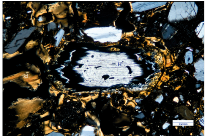
Abb. 1. Stark verwitterte Hornblende (H) mit ursprünglicher Tonanlagerung (cl) und Hämatite (He), fotografiert unter gekreuzten Polarisatoren.
