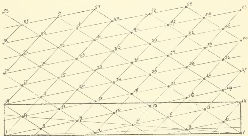
Fig. 41, Divergenz \frac{5}{13} .
