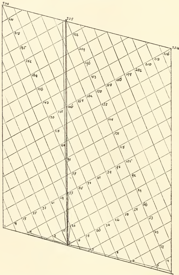
Fig. 50, Divergenz ^{69}/_{233} .
