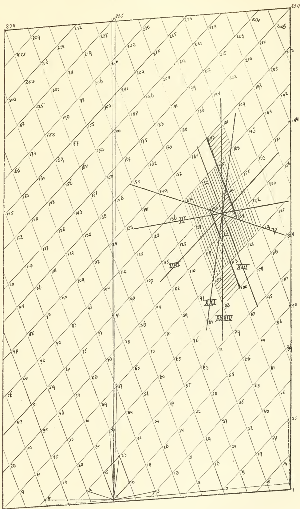
Fig. 48, Divergenz ^{89}/_{233} .
