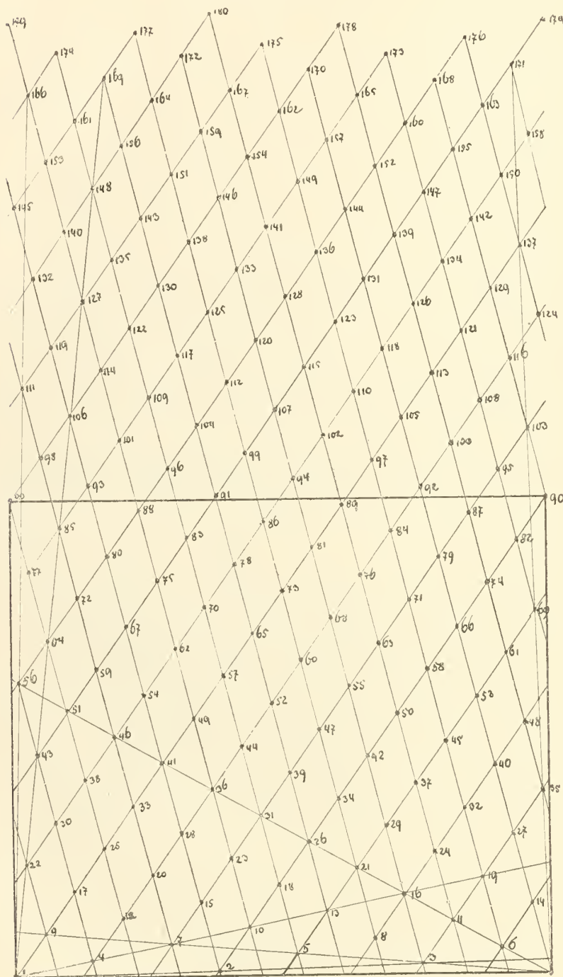
Fig. 45, Divergenz \frac{34}{89} .
