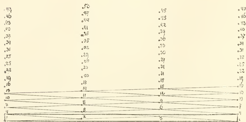
Fig. 39, Divergenz \frac{2}{5} .
