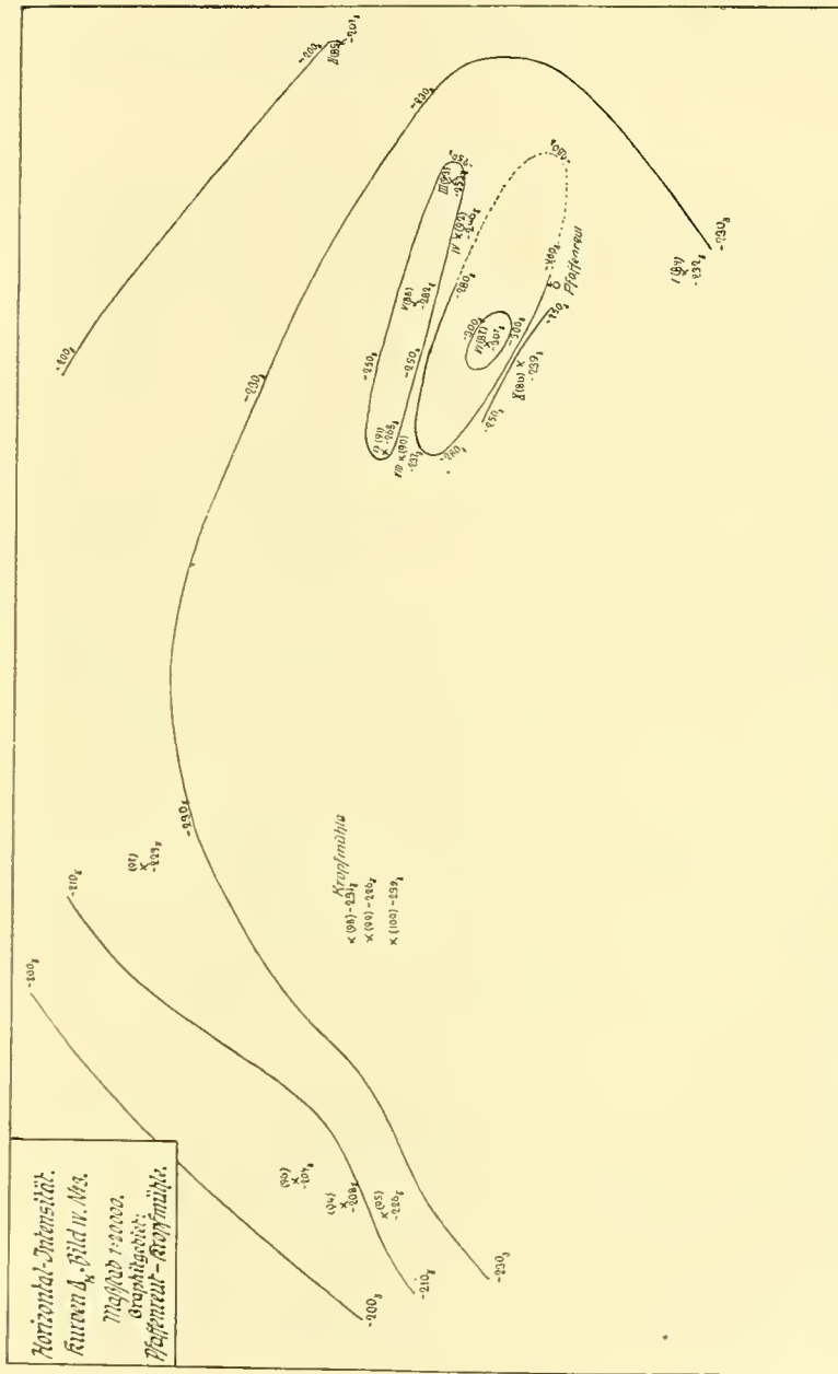
Bild IV. No. 3. Graphitgebiet. Horizontalintensität. Verlauf der \Delta_H -Kurven.
