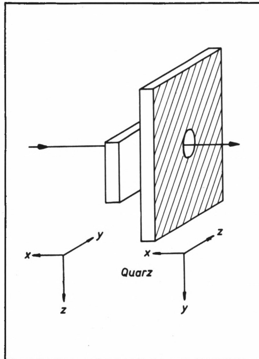
19. Lichtmodulation und schwingende Quarzkristalle nach Tavil.
