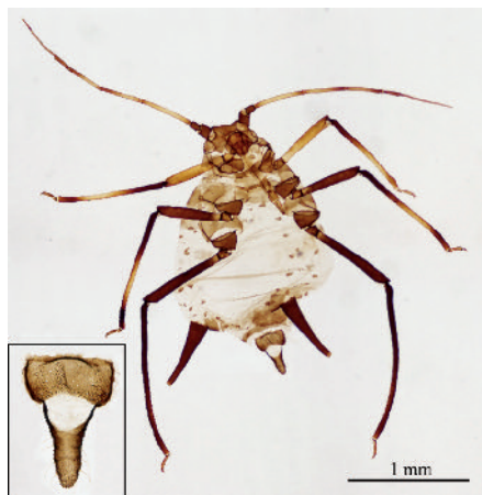
Sl. 4: Aphis illinoisensis – mikroskopski preparat nekrilate viviparne samice (v okvirju povečan repek – cauda)
