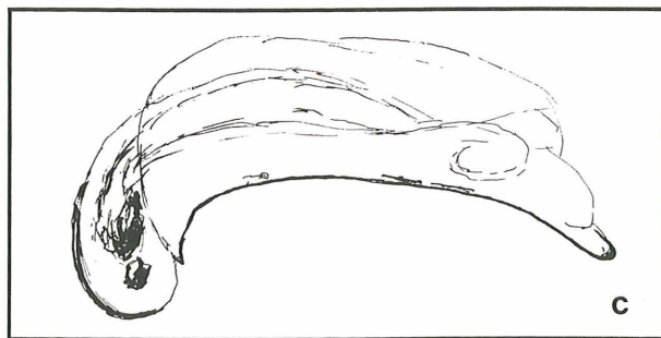
Abb. 3: Bembidion (Peryphanes) lafertei Jaqu. du Val; a) habitus, b) Augenwö Halsschildskizze, c) Aedoeagus
