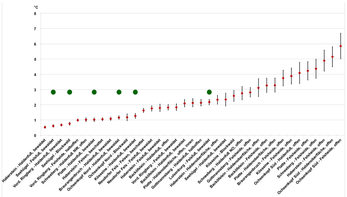
Abb. 6: Spanne \Delta t^{\circ}\text{C} des mittleren Temperaturmaximums und -minimums im Projektgebiet (Vertrauensbereich 95%, N=365). ● = Vorkommen von Leistus piceus .
