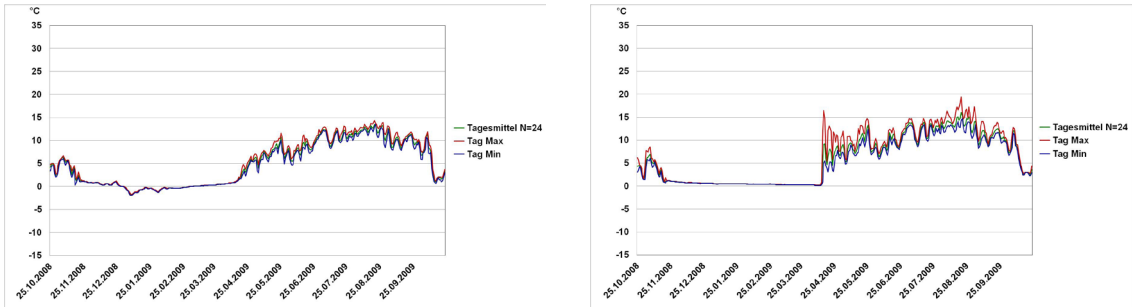
Abb. 5: Tagesmittel im Jahresverlauf im Untersuchungsgebiet Seehügel (Blockwald – links) und Backköfele (Haldenfuß, bewaldet).
