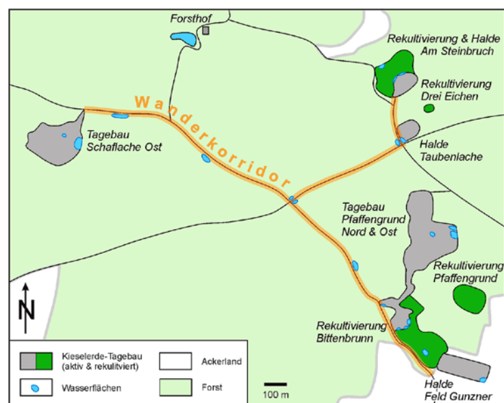
Abb. 3: Ausschnitt des Tagebaureals am Hainberg bei Neuburg an der Donau (nach LANDESAMT 2006). Um die Biotope und Wasserflächen in den Tagebauen, Halden und Rekultivierungen zu vernetzen, wurden entlang der Fahrwege kleine Wasserflächen angelegt. Diese können von Amphibien als Wanderkorridore (orange Markierung) genutzt werden.
