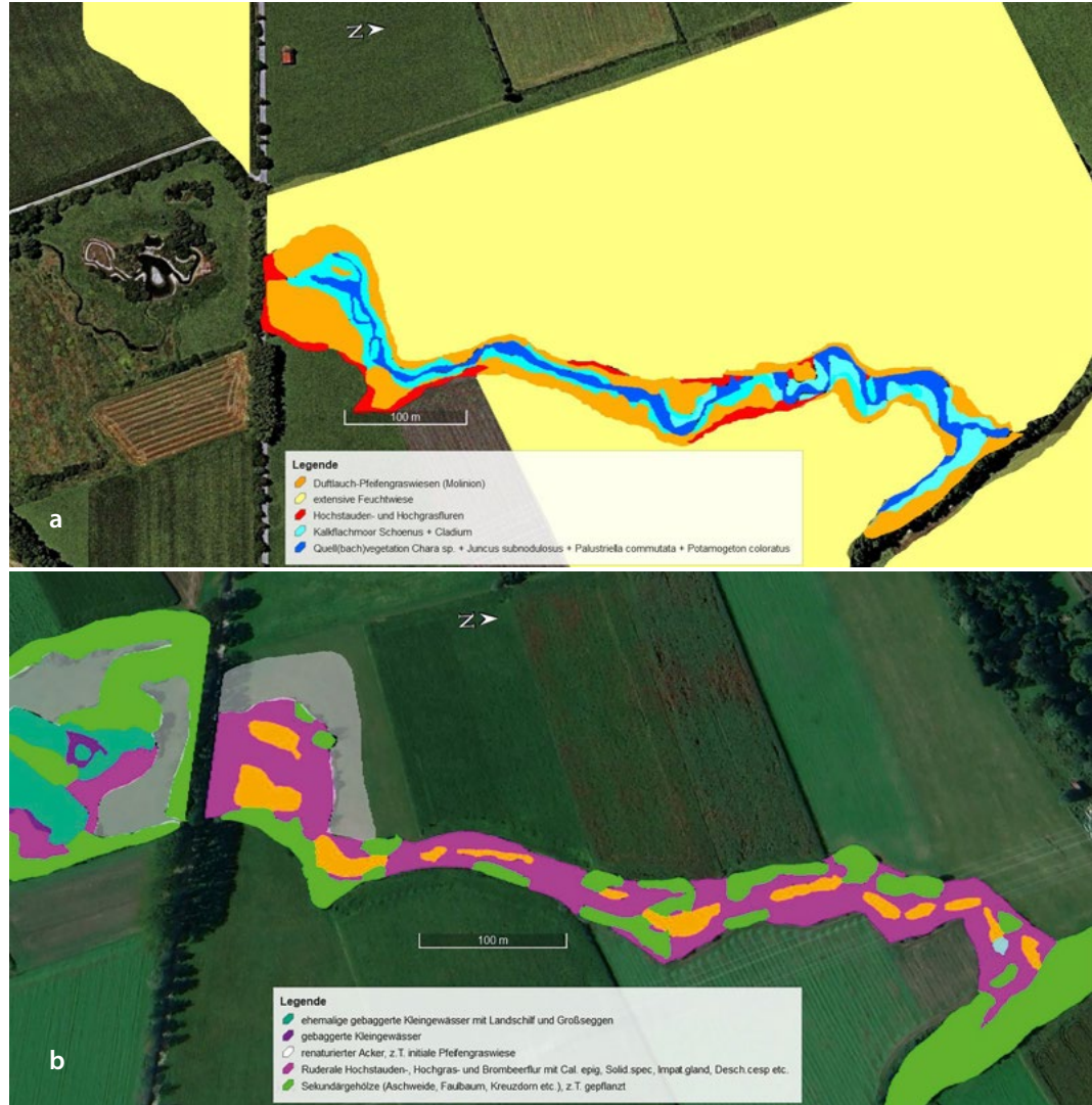
Abbildung 5a und b Kalkflachmoor Gfällach- ursprung NE Eicher- loh im südlichen Erdinger Moos 1962 (oben) und 2020 (unten; Karten: Alfred Ringler).
