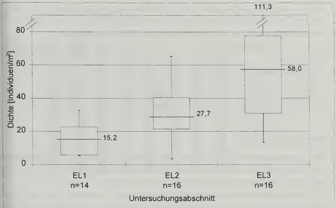
Abb. 3: Individuendichte (Individuen/m 2 ) der echten Spinnen (Araneae) an den drei Untersuchungsabschnitten des Elbrighäuser (dargestellt in "Box-and-Whisker-Plots" (Spannbreite, 1. und 3. Quartil, Median, n= Anzahl der untersuchten Schotterbänke)
