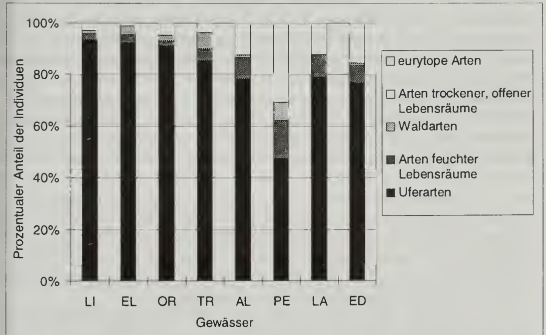
Abb. 5: Prozentualer Anteil der Individuen an den ökologischen Typen (Einordnung nach MAURER & HÄNGGI 1990)
