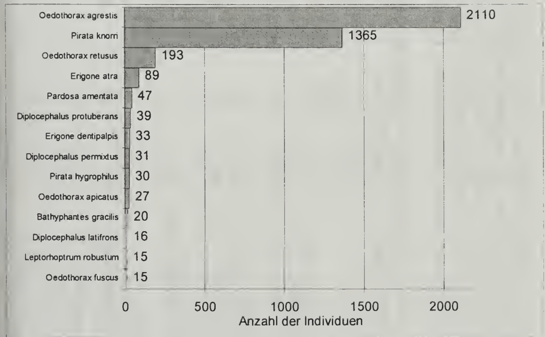
Abb. 2: Individuenanzahl der Spinnenarten, die insgesamt mit 15 oder mehr Individuen an der Wasserlinie nachgewiesen wurden
