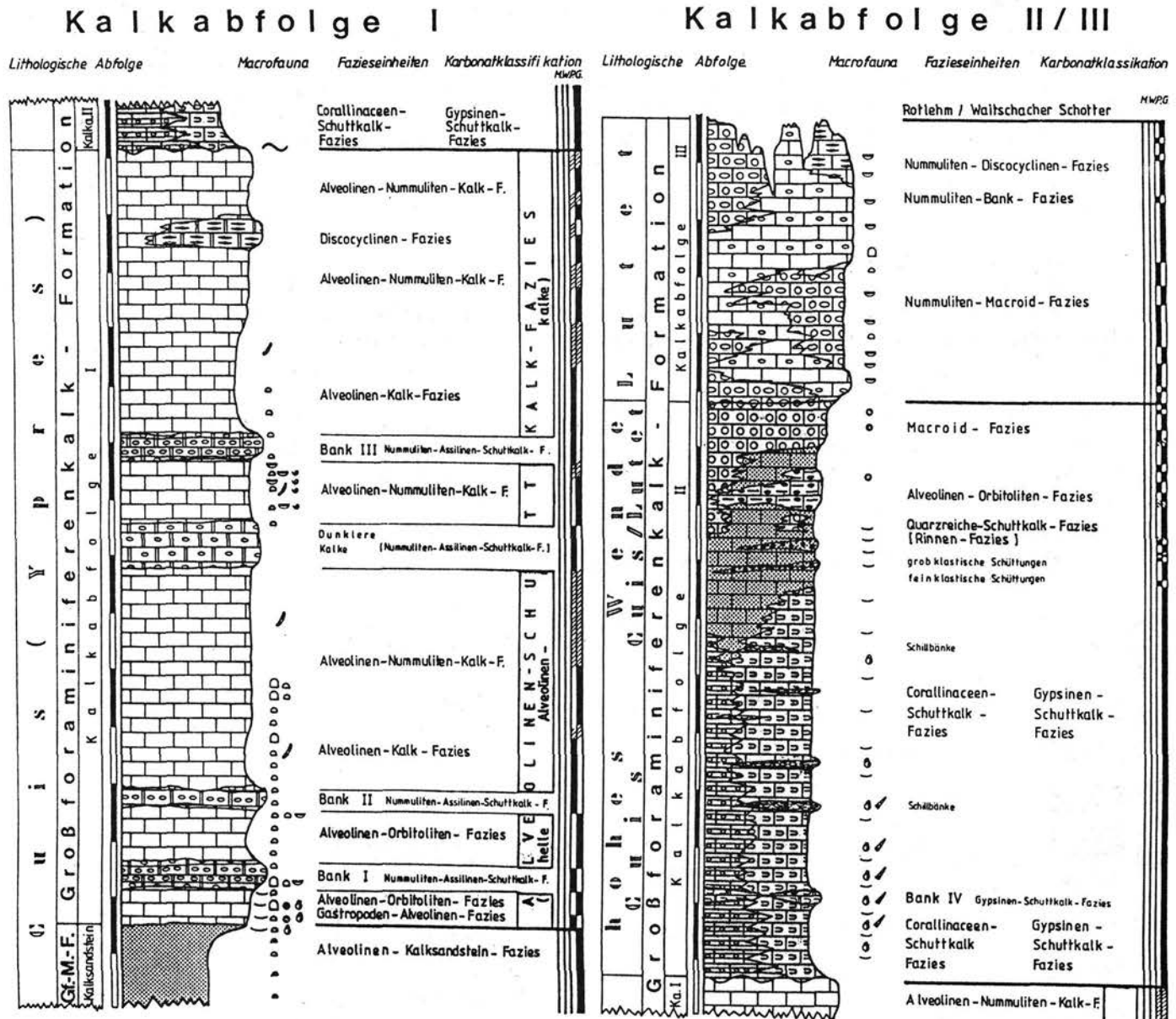
Abb. 3. Sedimentologie und Mikrofaziestypen der Großforaminiferenkalk-Formation des Sittenberges. Legende siehe Abb. 4.
