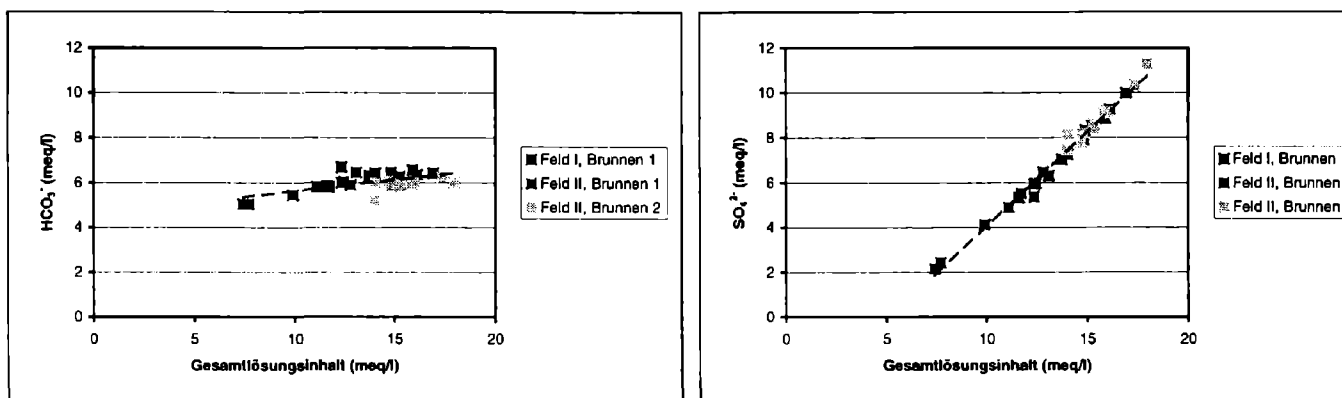
Abb. 8: Diagramm HCO 3 - gegen Gesamtlösungsinhalt
