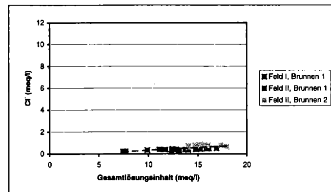
Abb. 7: Diagramm \text{Cl}^- gegen Gesamtlösungsinhalt
