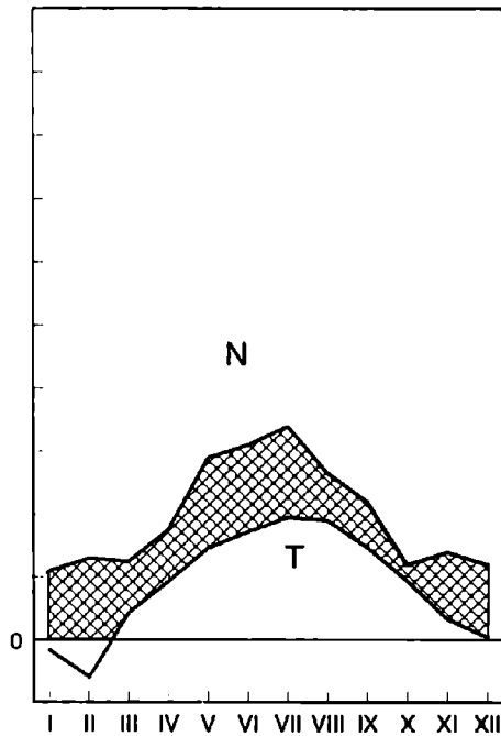
Abb. 2: Klimadiagramm zur Meßstelle Retz
