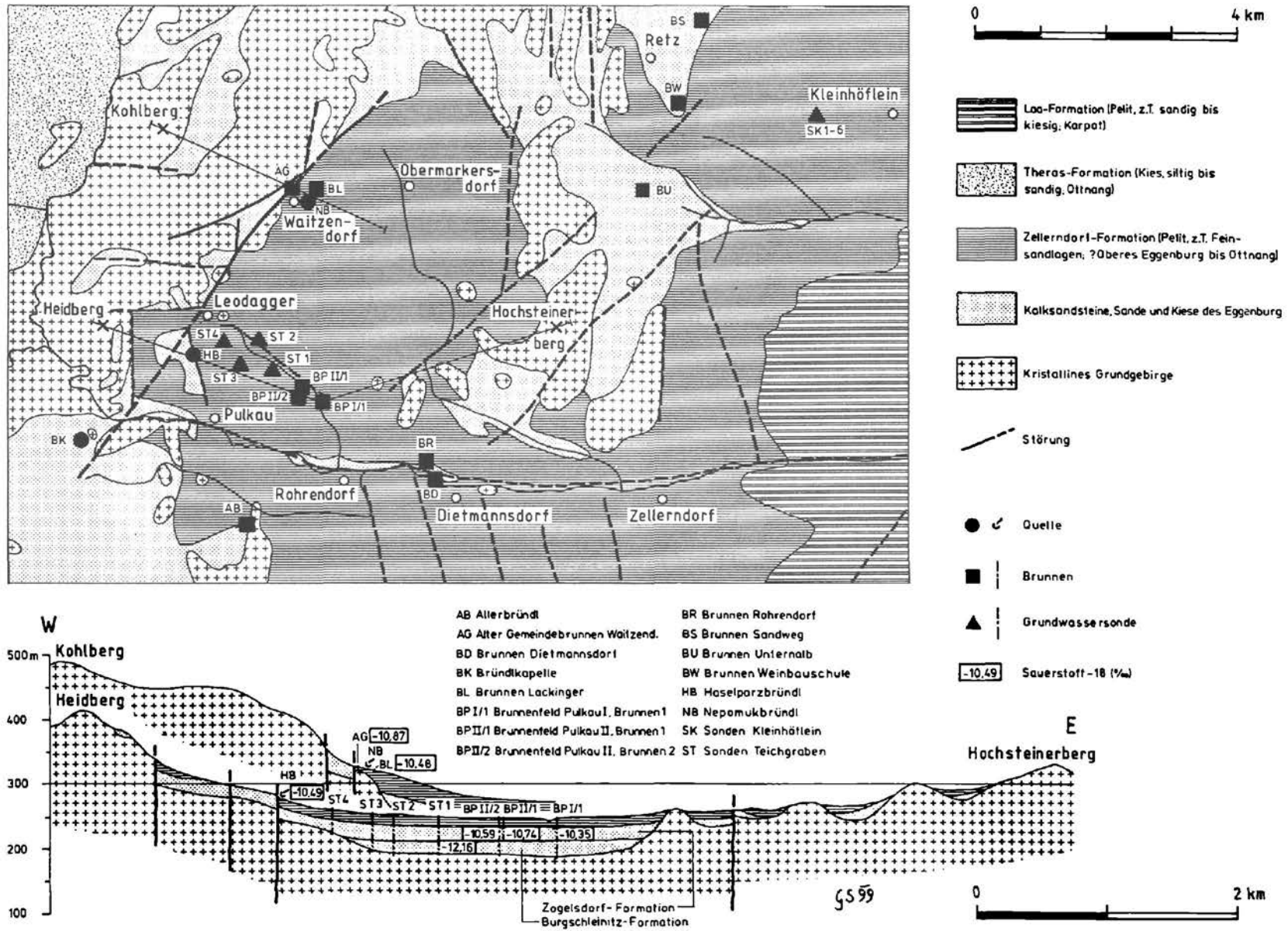
Abb. 1: Hydrogeologische Übersichtskarte des Obermarkersdorfer Beckens und seiner Umgebung; bei den im Profil enthaltenen \delta^{18}\text{O} -Werten handelt es sich um Mittelwerte der zum Bearbeitungszeitpunkt zur Verfügung stehenden Meßdaten.
