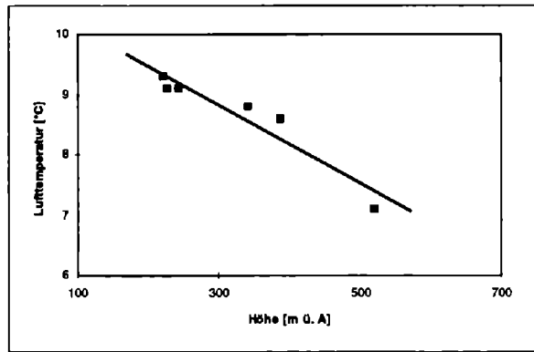
Abb. 5: Temperaturabnahme mit Seehöhe im Arbeitsgebiet
