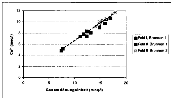
Abb. 4: Diagramm \text{Ca}^{2+} gegen Gesamtlösungsinhalt
