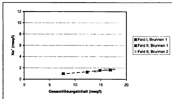
Abb. 6: Diagramm \text{Na}^+ gegen Gesamtlösungsinhalt
