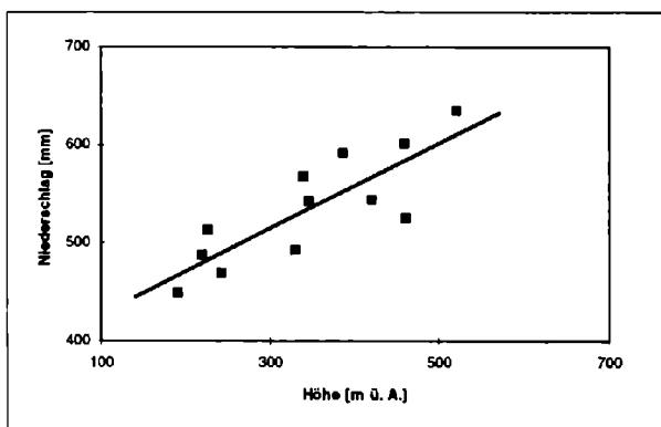
Abb. 4: Niederschlagszunahme mit Seehöhe im Arbeitsgebiet
