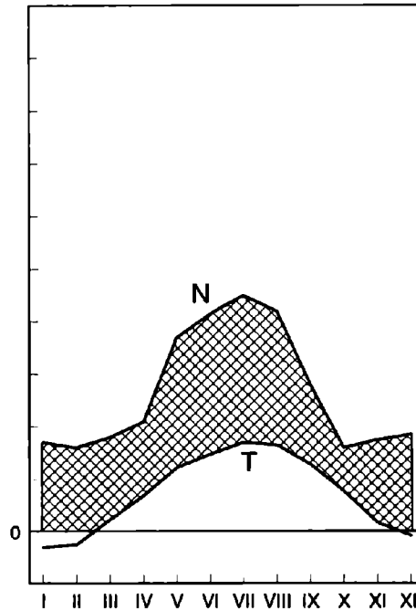
Abb. 3: Klimadiagramm zur Meßstelle Japons
