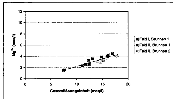
Abb. 5: Diagramm \text{Mg}^{2+} gegen Gesamtlösungsinhalt
