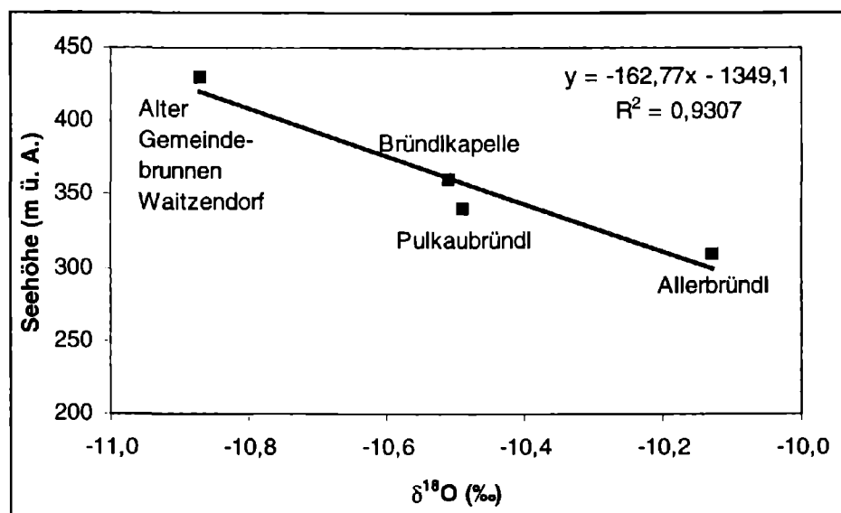
Abb. 1: Höheneffekt bei ^{18}\text{O} unter Verwendung der Daten der Meßstellen in Tab. 1: das unübliche Resultat von -0,6 \text{ ‰}/100 \text{ m} ist offensichtlich auf Klima- bzw. Vegetationseffekte zurückzuführen.
