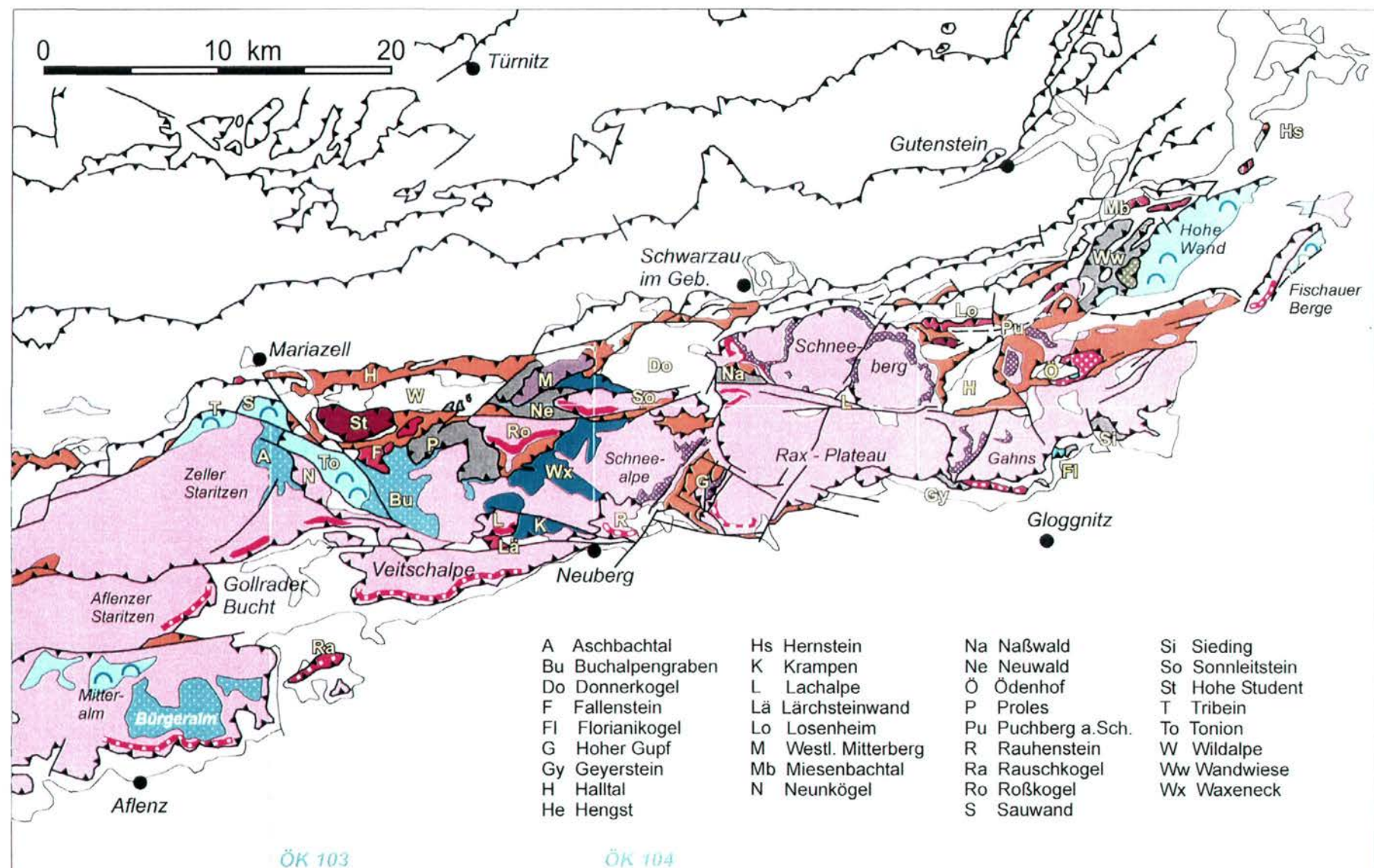
Abb. 2: Tektonisch - fazielle Übersicht des Juvavikums der östlichen Kalkhochalpen (schematisch); Farblegende siehe Abb.2
