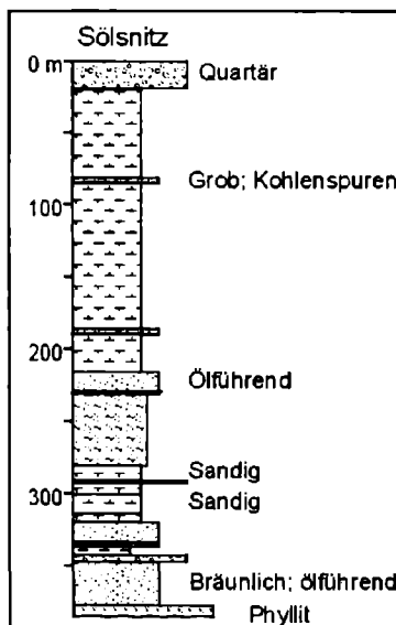
Abb. 6. Profil der Bohrung Sölsnitz (PETRASCHECK, 1922/25). Legende siehe Abb. 3.
