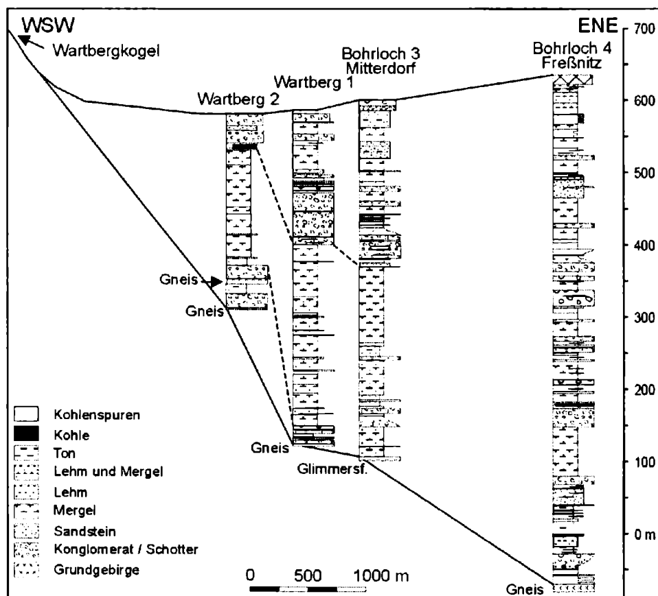
Abb. 3. Profile von Tiefbohrungen im oberen Mürztal nach unveröffentlichten Bohrprotokollen.
