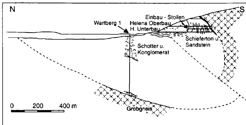
Abb. 4. N-S Profil durch den ehemaligen Bergbau Wartberg (modifiziert nach PETRASCHECK, 1922/25).
