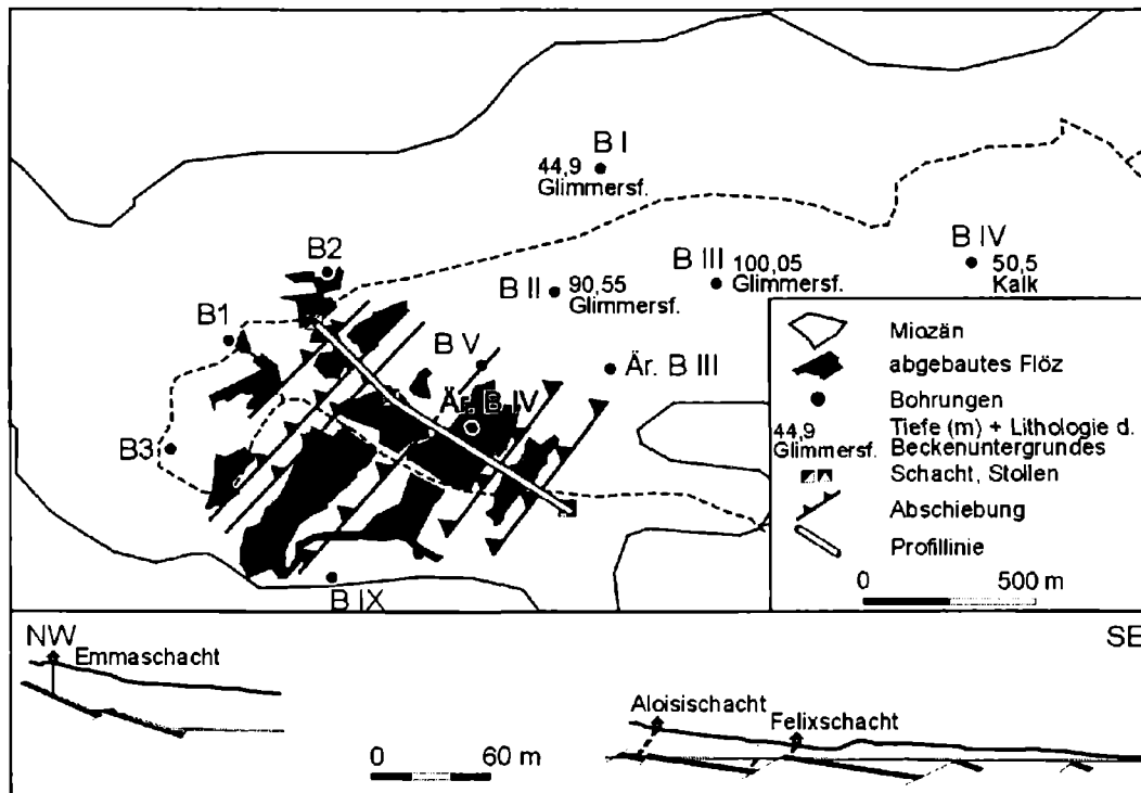
Abb. 5. Lageplan des Parschluger Bergbaus und NW-SE Profil (nach WEBER & WEISS, 1983).
