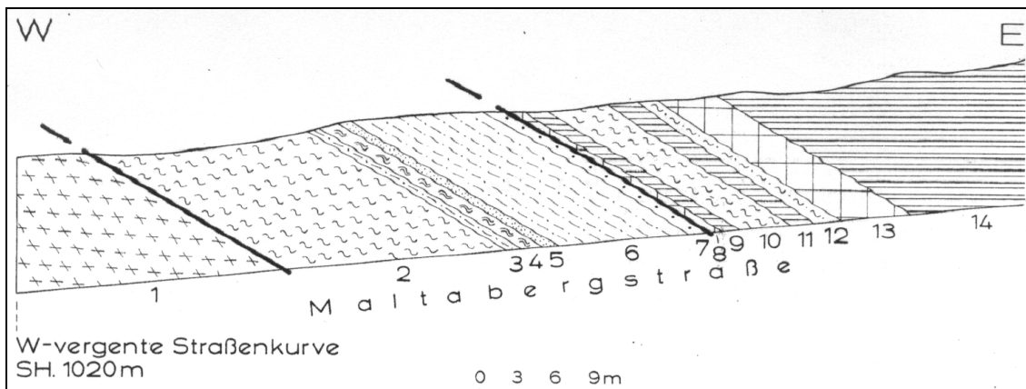
Abb. 3: Profil durch die basalen Teile der peripheren Schieferhülle längs der Maltabergstraße. Sockel des Maltaberges, Sh. 1020 bis 1030 m (nach Ch. EXNER [1980]; tektonische Grenzen ergänzt).
