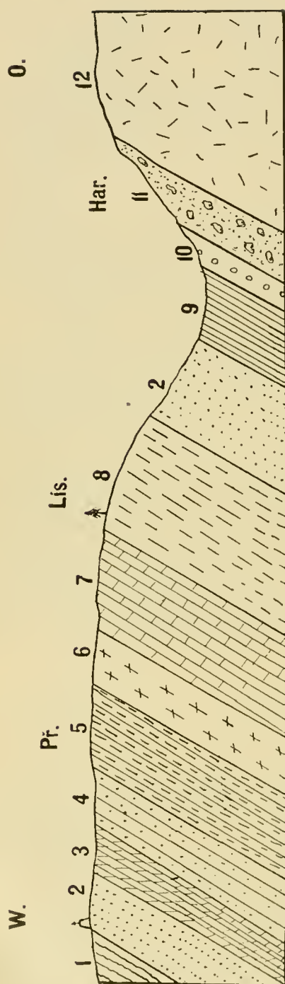
Fig. 11. Profil längst des Weges „Přínice“ bei Alt-Paka nach Prof. Dr. A. Frič.
