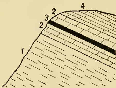
Fig. 7. Profil bei dem Viadukt der Semil-Liebstädter Eisenbahn (nör. von Želechov.)
