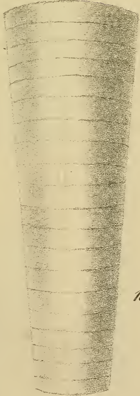
18. Orthoceras imbricatum Wahlb. 19. O. Hagenowii Boll.
