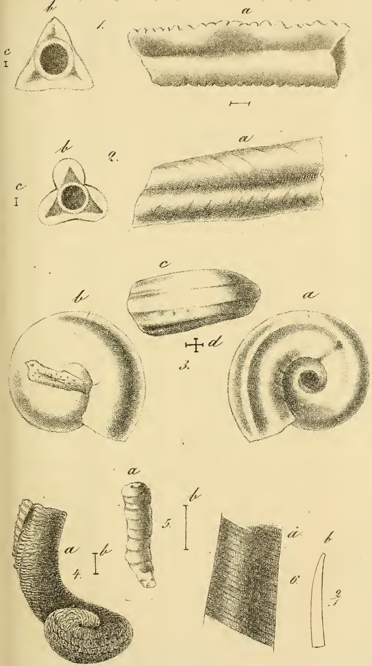
1. Serpula serrata Boll. 2. S. Huthii Boll. 3. S. bicarinata Boll. 4. S. asperima Boll. 5. S. cylindrica Boll. — 6. Dentalium tenuistriatum Boll.
