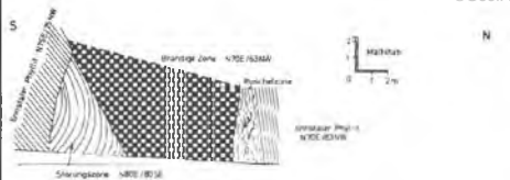
Detallaufnahme beim 8 Wehr im Nieder-Obblarner Graben
