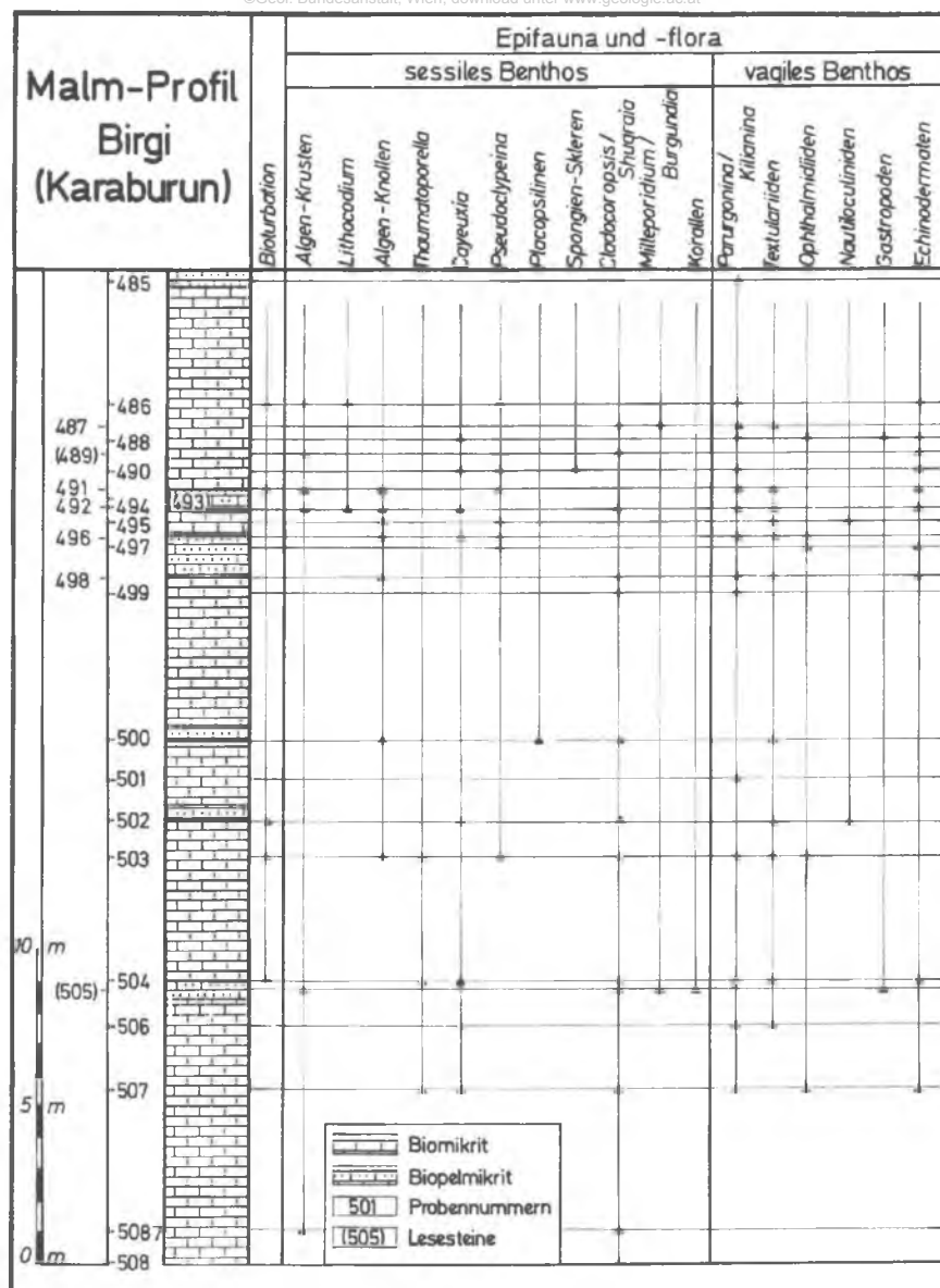
Abb. 1. Mikrofazies und Fossilverteilung im Malm-Profil von Birgi, Halbinsel Karaburun, W-Anatolien
