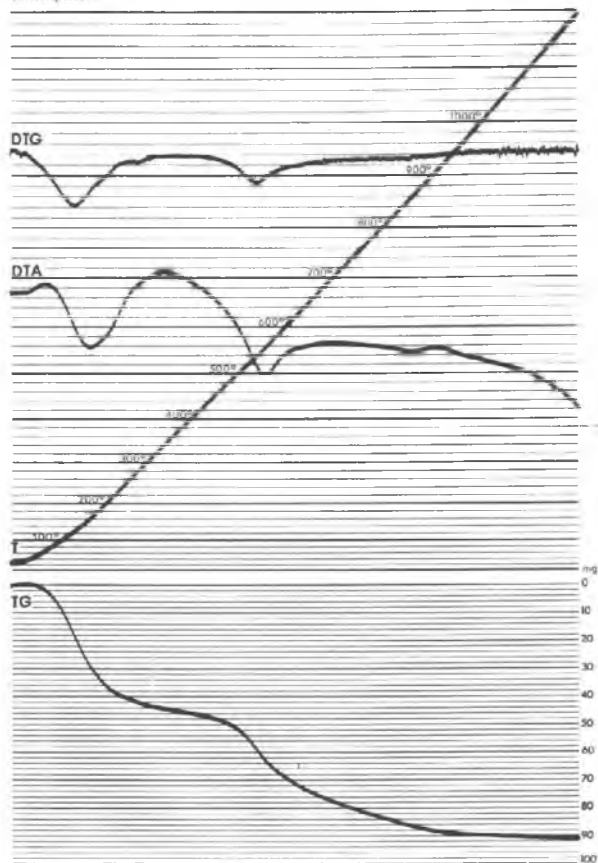
Abb. 1. Derivatographische Aufnahme (System ERDEY, F. PAULIK & J. PAULIK) eines sandig-tonigen Feinsedimentes aus der Würmterrasse in Graz, Brucknerstraße. — DTG = Differentialthermogravimetrische Kurve. DTA = Differentialthermoanalytische Kurve. T = Temperaturkurve. TG = Thermogravimetrische Kurve. Einwaage = 1,0 g.
