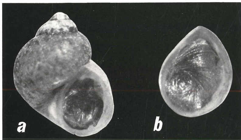
Fig. 2. a) Sadleriana fluminensis (KÜSTER) des environs de Milan; b) détail de l'opercule. (Phot. GIROD).
