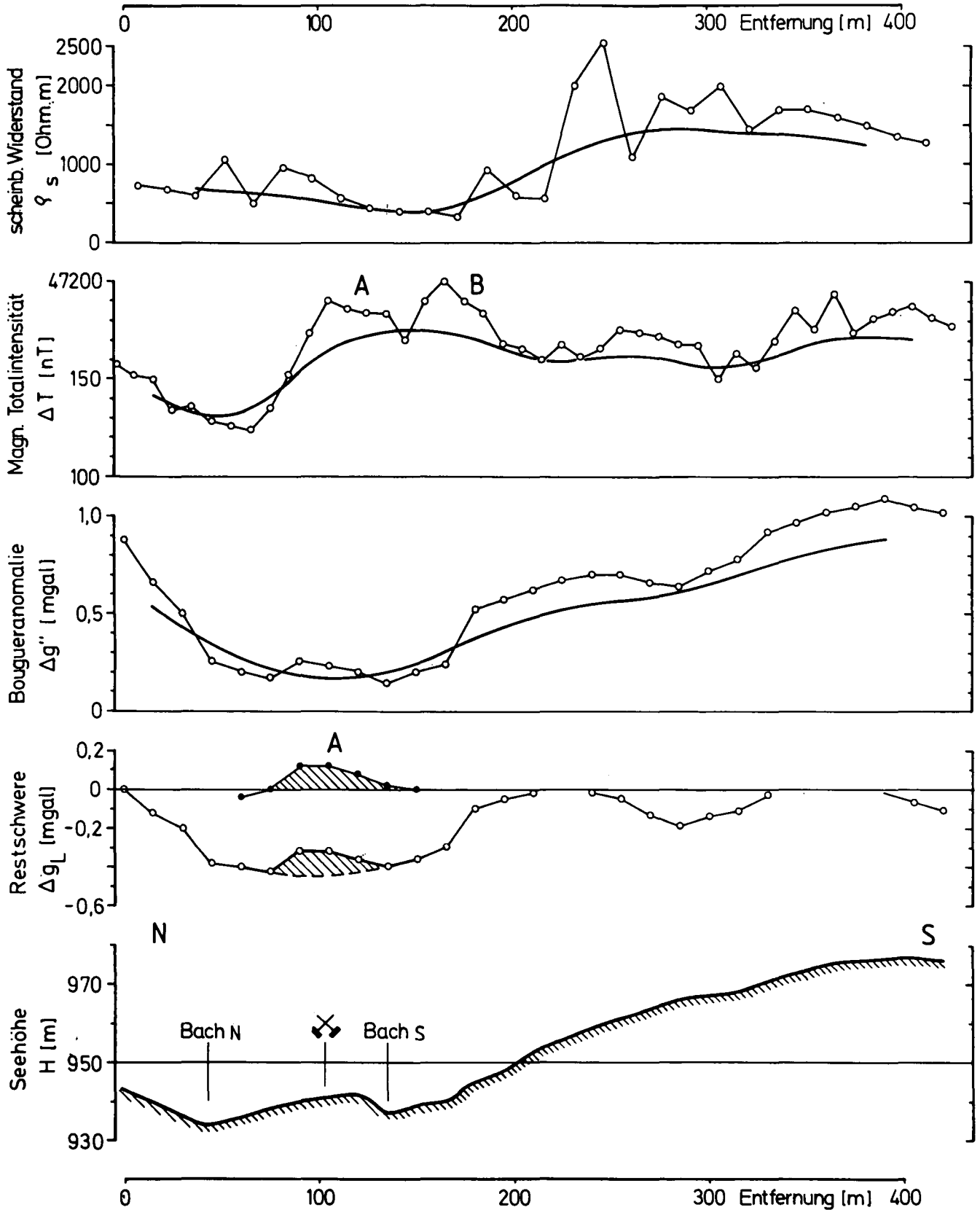
Abb. 3. Geoelektrische, magnetische und gravimetrische Meßergebnisse für das Testprofil EI.
