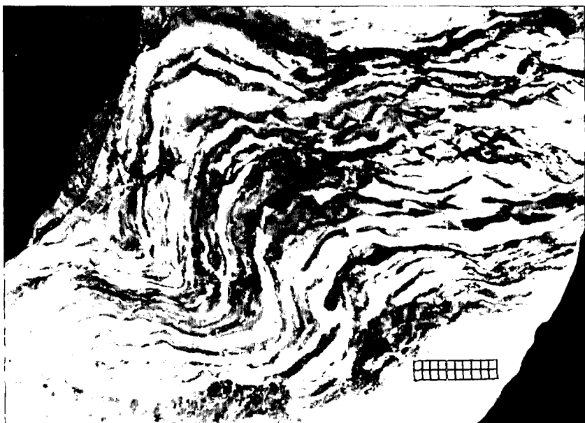
Abb. 9. Stetige fältelnde Deformation in verschiedenen Entwicklungsstadien des polymineralischen "Schiefererzes" (Quarz-Sericit-Sideritphylit). Maßstab: mm-Papier.
