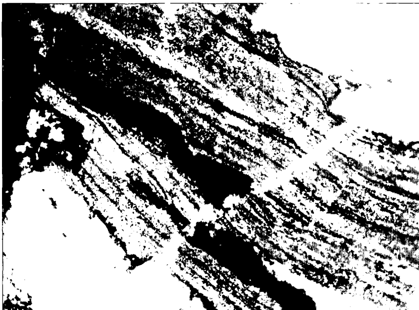
Abb. 6. Mikrokristalliner polymineralischer Ferrodolomit/Mesitinspat-Lutit mit schräggeschichtetem Teilbereich als Verdrängungsrelikt zwischen grobkristallinen Sideritlagen, welche durch einen, mit Siderit zementierten Haarriß verbunden sind. Sekundäre Limonitlagen schwarz. Dünnschliff, 1 Nicol, natürl. Gr. 1.44x0.94 mm.
