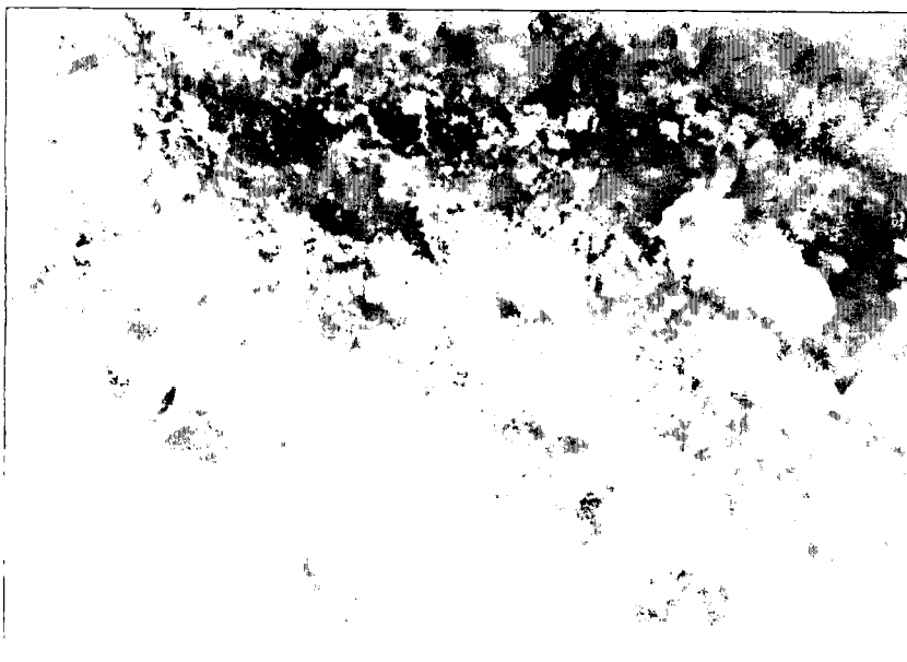
Abb. 5. Mikrokrystalline Ferrodolomit/Mesitinspat-Laminae sind durch Sammelkristallisation von Siderit zerstört. Polierter Anschliff, Nicolsx, natürl. Gr. 0.54x0.36 mm.
