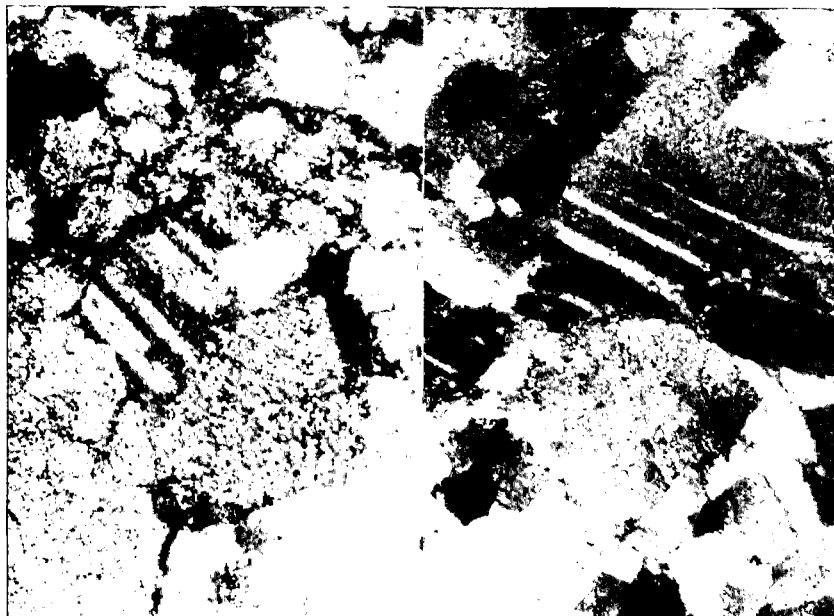
Abb. 11. Undulöse Auslöschung und seltene Druckzwillingbildung als Folge nachkristalliner intragranularer Gitterdeformation in alternierenden, unterschiedlich grobkristallinen Sideritlagen. Dünnschliff, Nicols +, natürl. Gr. linkes Bild 2.2x1.7 mm, rechtes Bild 0.94x0.63 mm.
