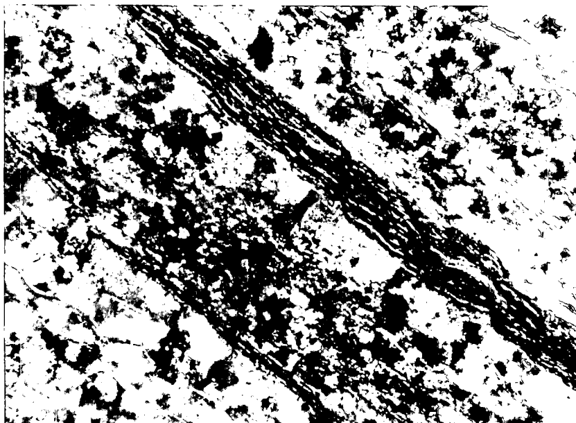
Abb. 7. Feinlagenbau durch laminaren Korngrößenwechsel des Siderits, durch Sericitzwischenschichten und Quarzeinschaltungen. Aus Sideriterzlager Typ "Schiefererz". Dünnschliff, Nicols +, natürl. Gr. 3.3x 2.1 mm.
