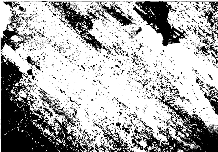
Abb. 13: Abbildungskristallisation: Mikrokristalliner Ankerit/Mesitinspat-Lutit wird von Sideritblasten selektiv verdrängt. Polierter Anschliff, Nicols x; natürl. Gr. 2.4x1.6 mm.
