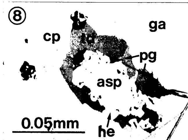
Abb. 8. Arsenopyritfragment (asp) als Einschuß in Galenit (ga), umwachsen von Chalkopyrit (cp), Fahlerz (td), Pyrraryrit (pg) und Hessit (he). Öl, Nicols ||.
