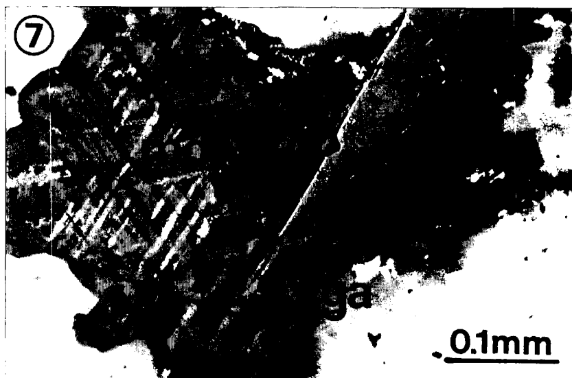
Abb. 7. Ehemaliger Mischkristall von Pb und AgBiS 2 zerfällt in Matildit (md) und Galenit (ga), daneben Pyrit (py). Foto: W.H. PAAR. Öl, Nicols x.
