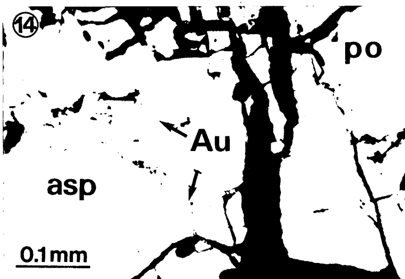
Abb. 14. Ged. Gold (Au) als Einschluß und rißfüllend in Arsenopyrit (asp), daneben Pyrrhotin (po). Öl, Nicols ||.
