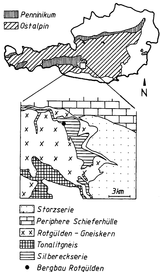
Abb. 1. Geologische Übersicht der Silbereckserie und der Zentralgneise. Vereinfacht nach EXNER (1982).
