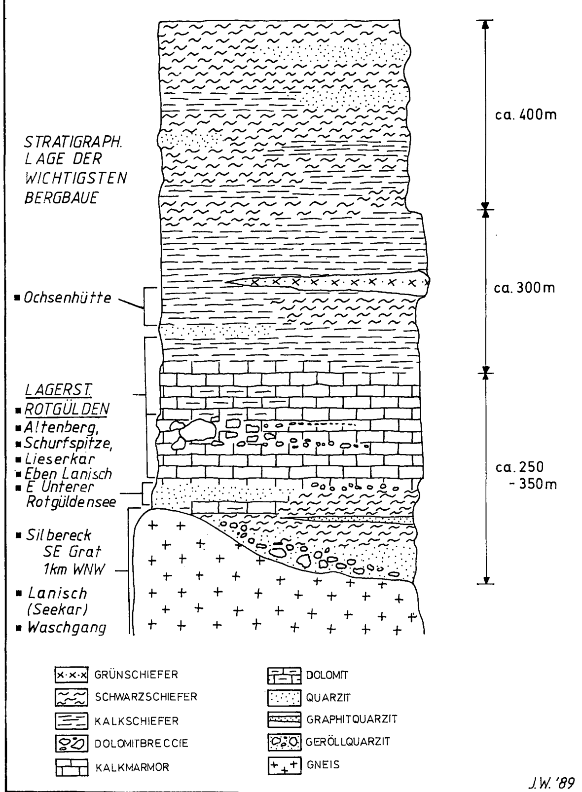
Abb. 3. Säulenprofil der Silbereckserie. Verändert nach J. KRUHL & H.P. STEYRER.
