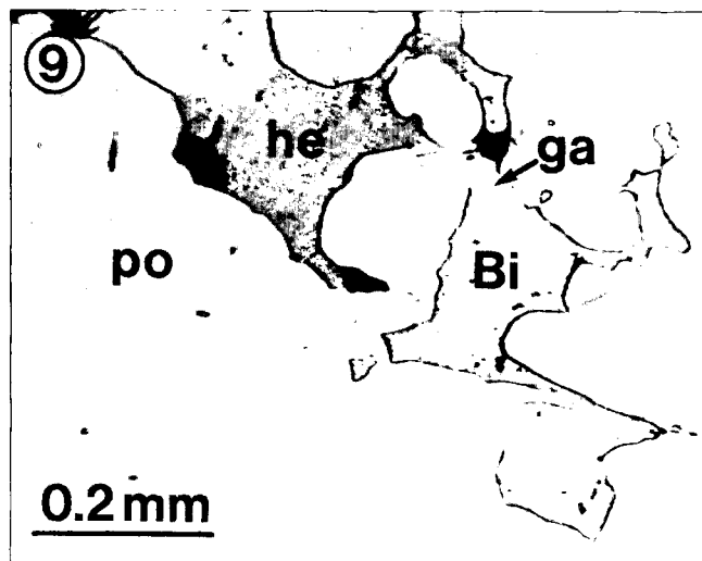
Abb. 9. Wismut (Bi) verwachsen mit Hessit (he) und Galenit (ga) als Einschuß in Pyrrhotin (po). Öl, Nicols ||.
