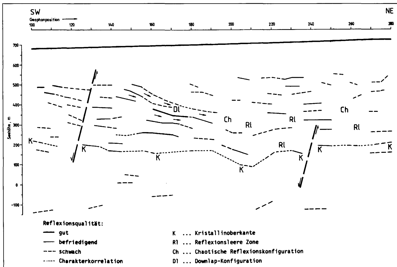
Abb. 5. Tiefenprofil GLB 2.
