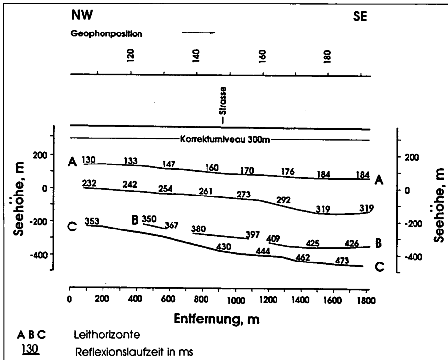
Abb. 6. Tiefenprofil HI8701 (Ausschnitt Geophonposition 100-193).
