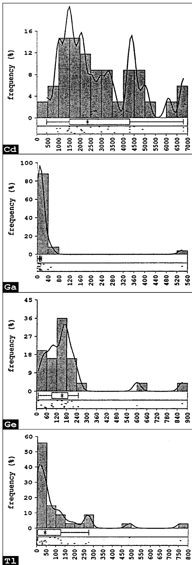
Abb. 3. Häufigkeitsverteilung von Cd, Ga, Ge und Tl in Sphaleritproben aus Lafatsch (n = 30).
