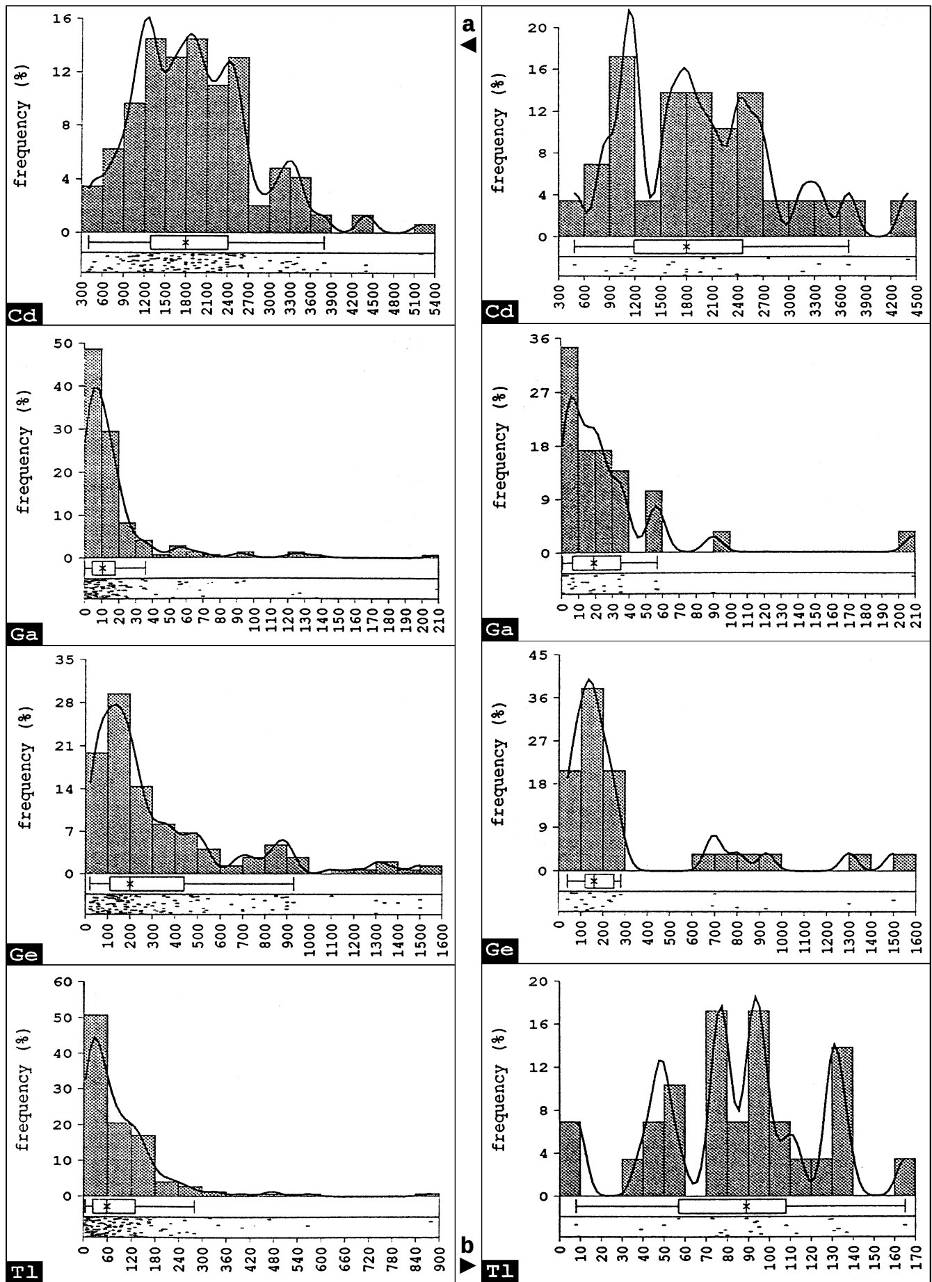
Abb. 2. Häufigkeitsverteilung von Cd, Ga, Ge und Tl in Sphaleritproben aus Bleiberg (a; N = 146) und aus dem Westen (b; N = 29).
