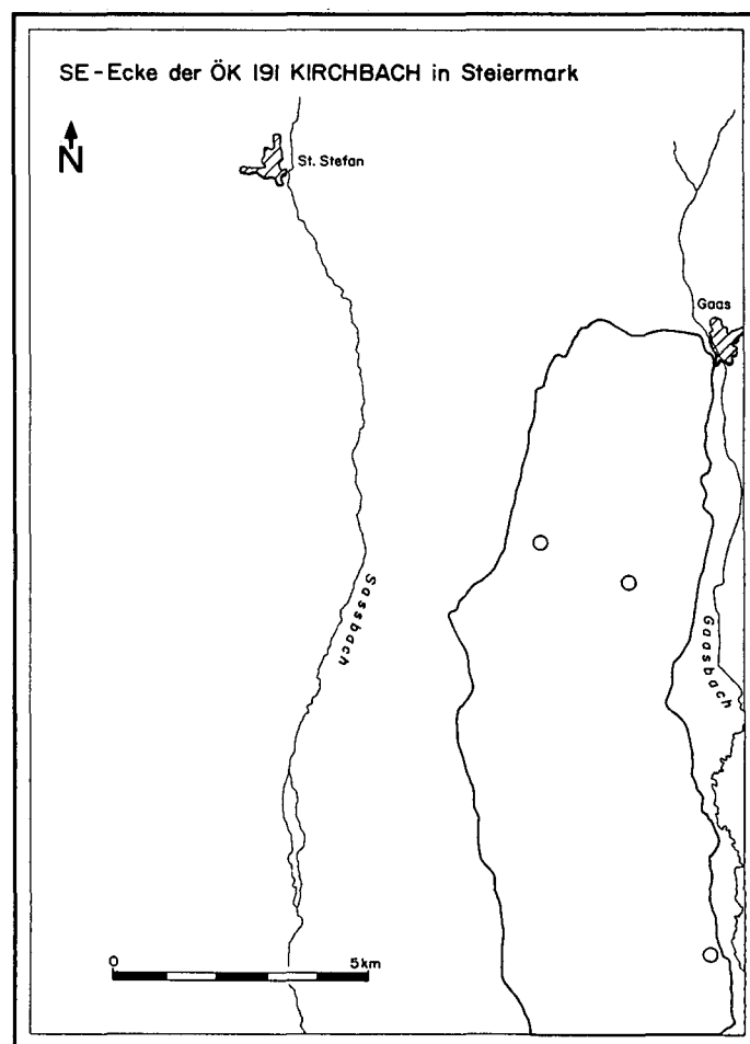
Abb. 2: Schematischer Lageplan des Kartierungsgebietes auf 1 : 10.000 auf ÖK-Blatt 191, Kirchbach i. Stmk. Vorrangige Hoffnungsgebiete für die Schotter/Kies-Gewinnung sind durch Kreise markiert.
