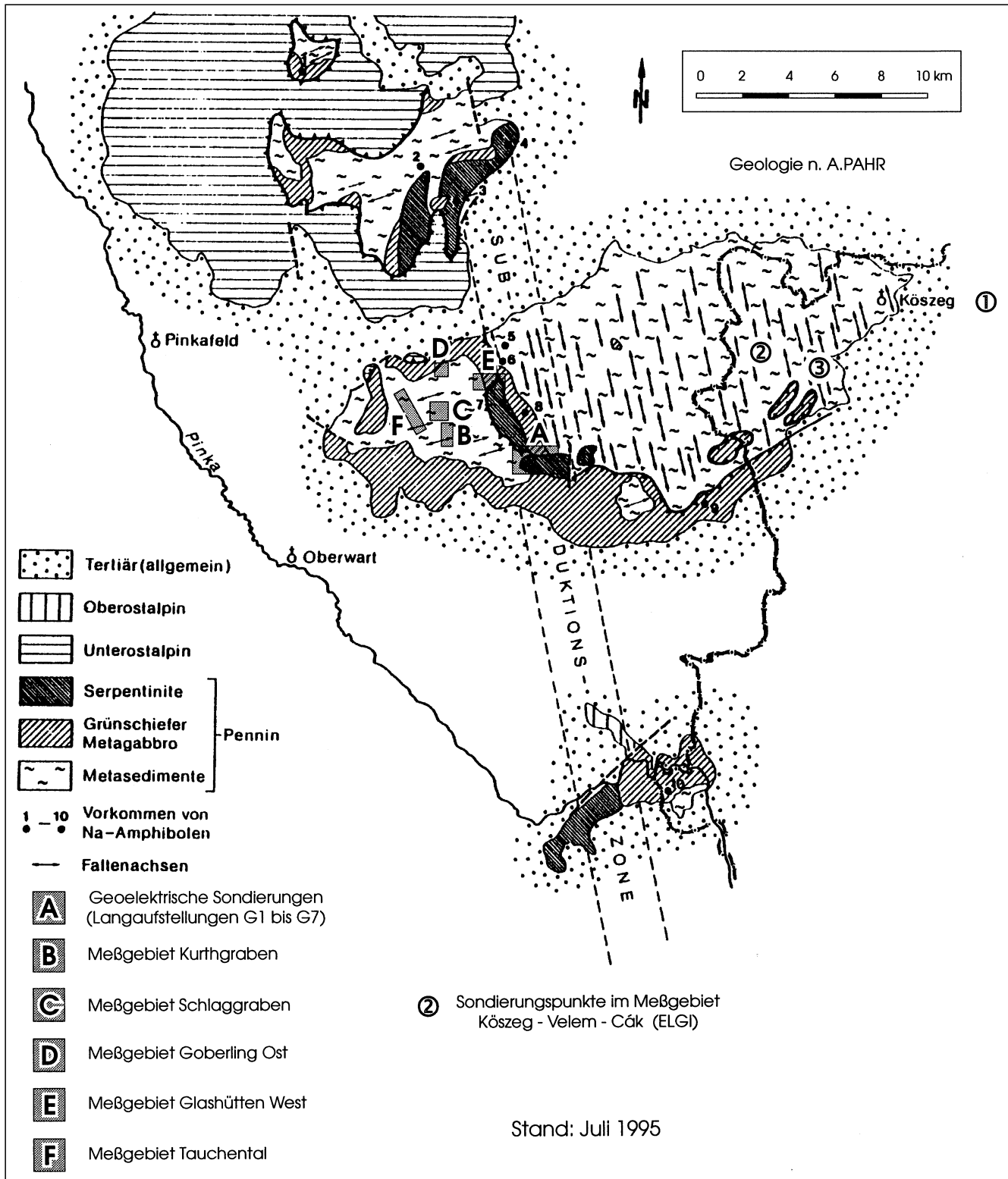
Abb. 1. Gesamtanlageplan mit Geologie.
