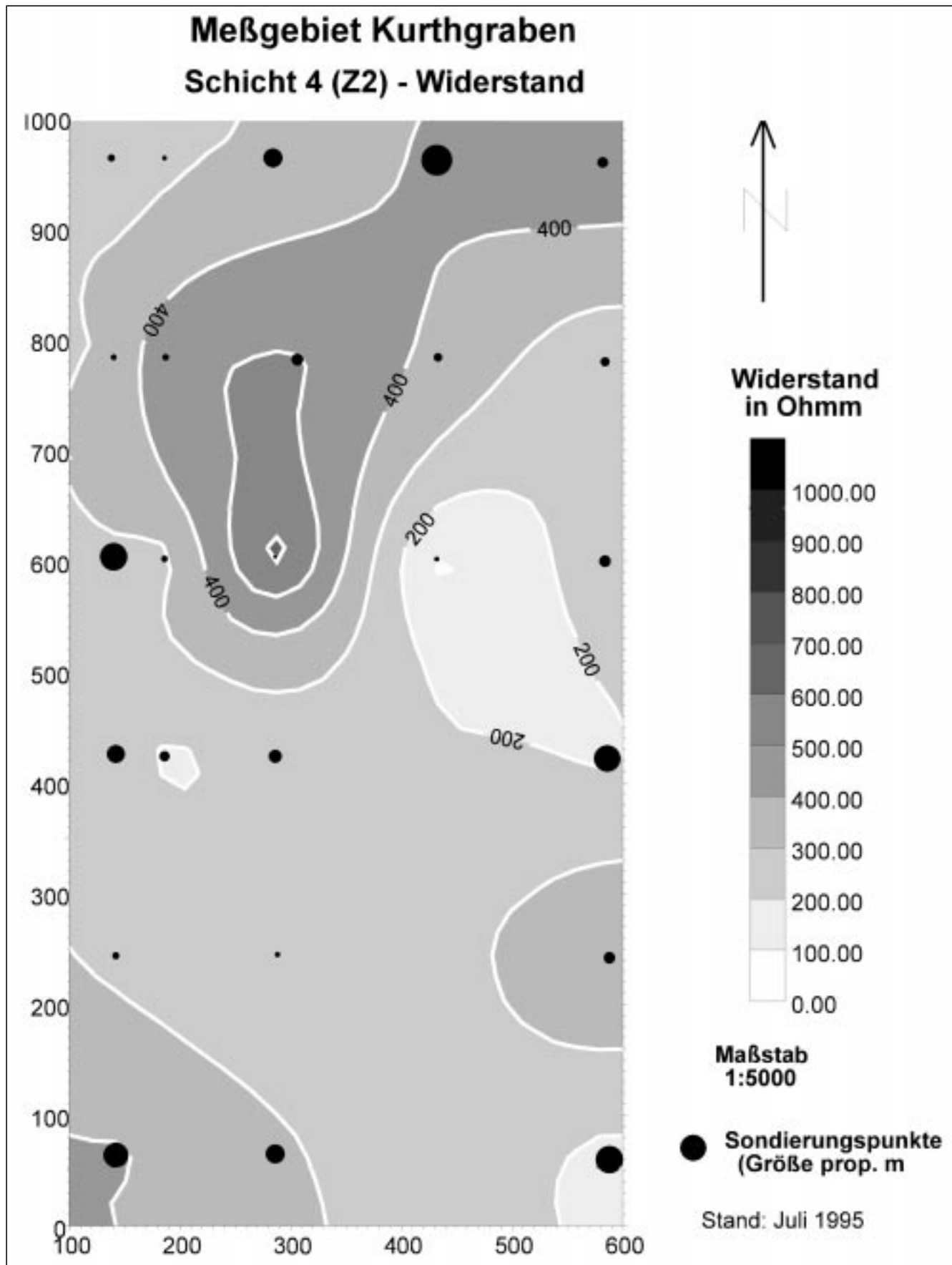
Abb. 8. Isoohmenkarte des \rho_4 -Horizontes (Z2) - Meßgebiet Kurthgraben.
