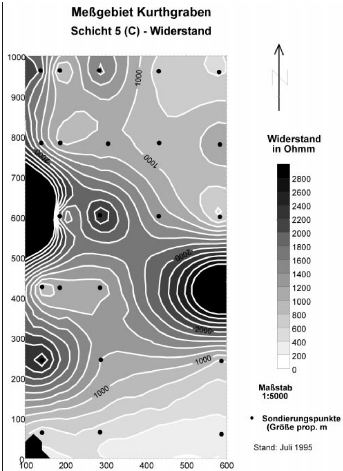
Abb. 9. Isohyetenkarte des \rho_5 -Horizontes (C) – Meßgebiet Kurthgraben.
