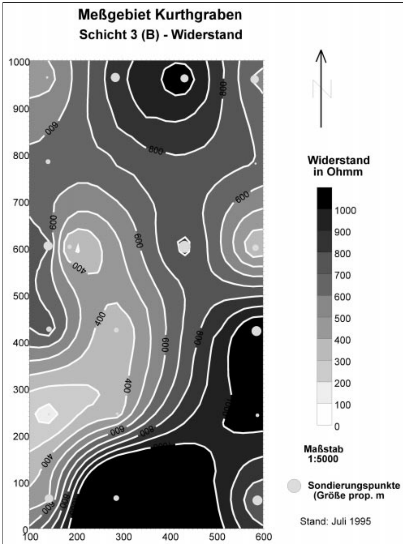
Abb. 7. Isohyetenkarte des \rho_3 -Horizontes (B) – Meßgebiet Kurthgraben.
