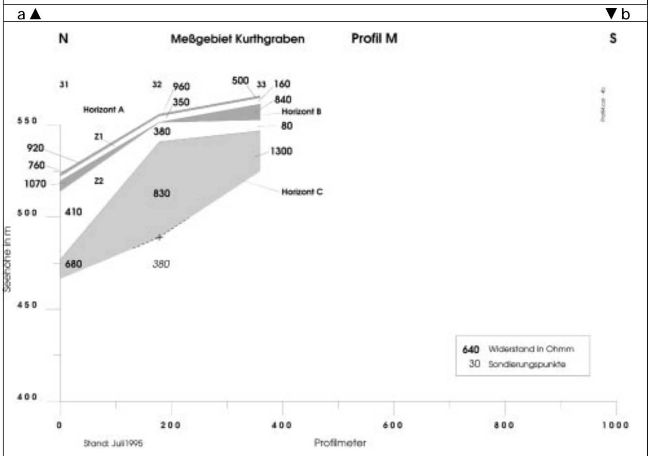
Abb. 4. Meßgebiet Kurthgraben: Geoelektrik-Profile I (a), M (b) und P (c; S. 20).
