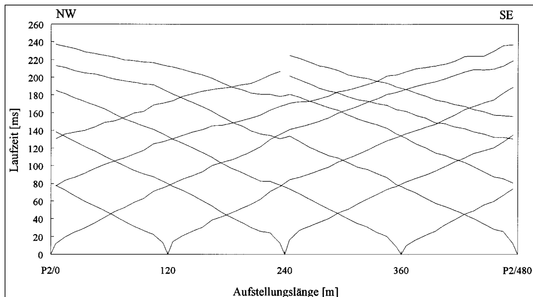
Abb. 3. Laufzeitkurven – Profil 2.
