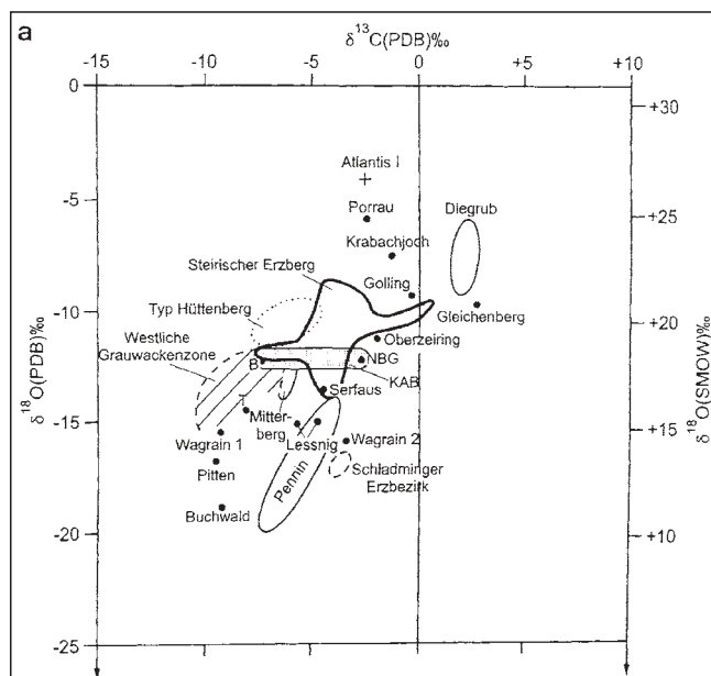
Abb. 25. \delta^{13}\text{C} vs. \delta^{18}\text{O} -Diagramm von Sideriten (beim Steirischen Erzberg auch von Ankeriten). KAB = Kalkalpenbasis; B = Bartholomäberg; NBB = Neuberg. Aus E. SCHRÖLL u. Mitarb. (1997; Lit. 266, 339).
