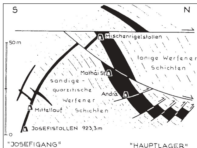
Abb. 22. Schematischer Saigerriss durch die Eisenspat-Ganglagerstätte Gollrad. Aus L. WEBER (1977; Lit. 335, 339).
