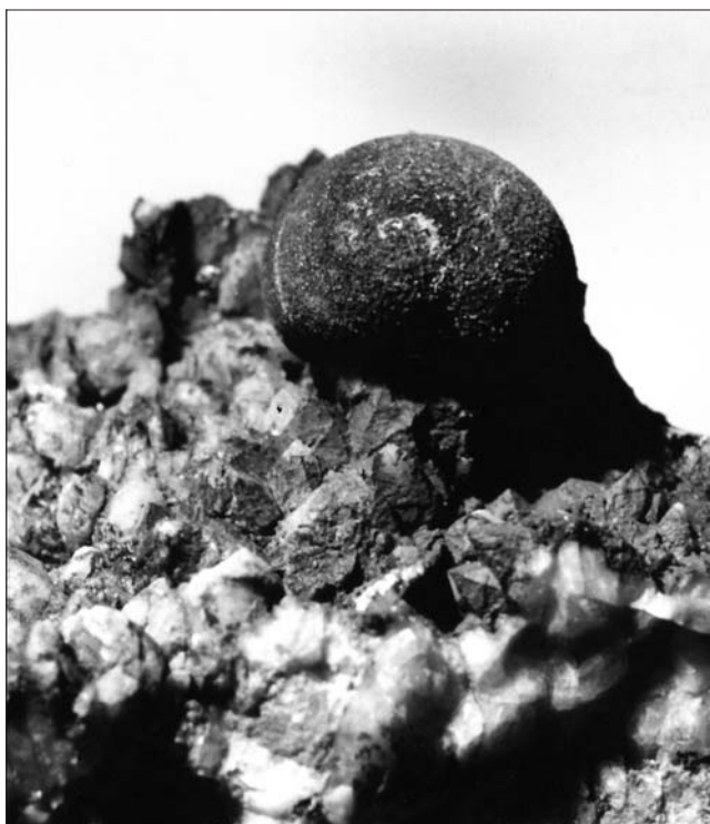
Abb. 44. Malachit Knappenberg. Kugeliges Aggregat, ca. 7 mm Durchmesser. Coll u. Foto K. WANER (1988).
