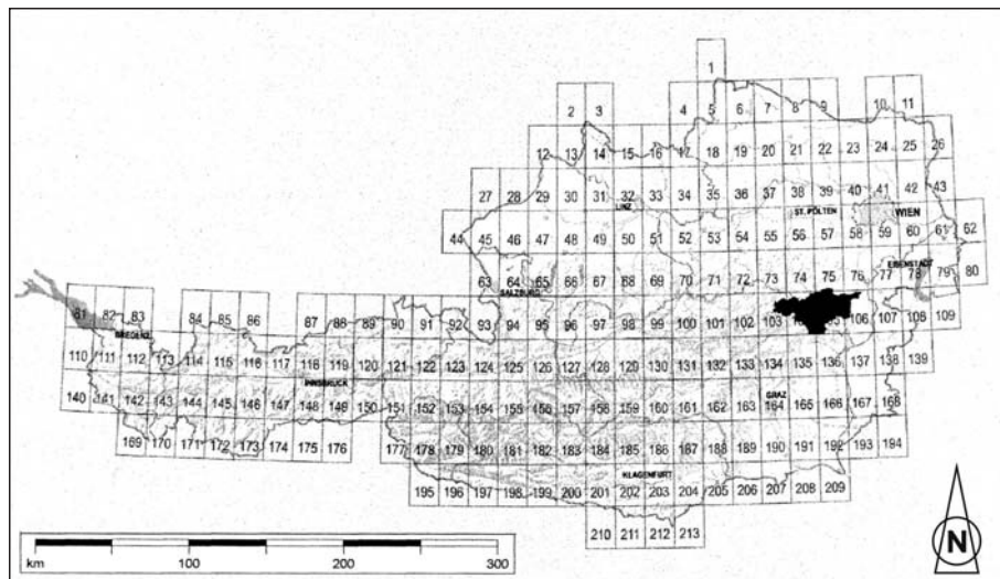
Abb. 1. Die Lage des Semmeringgebietes (ca. 900 km 2 ) im Bereich der Republik sterreich im Blattspiegel der K 50.
