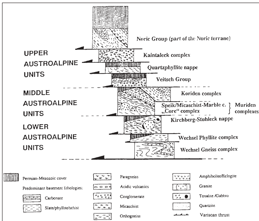
Abb. 9. Tectonostratigraphy of Austroalpine units exposed in the Eastern Alps. Die Grobgnesserie ist hier als Kirchberg- Stuhleck nappe bezeichnet.
