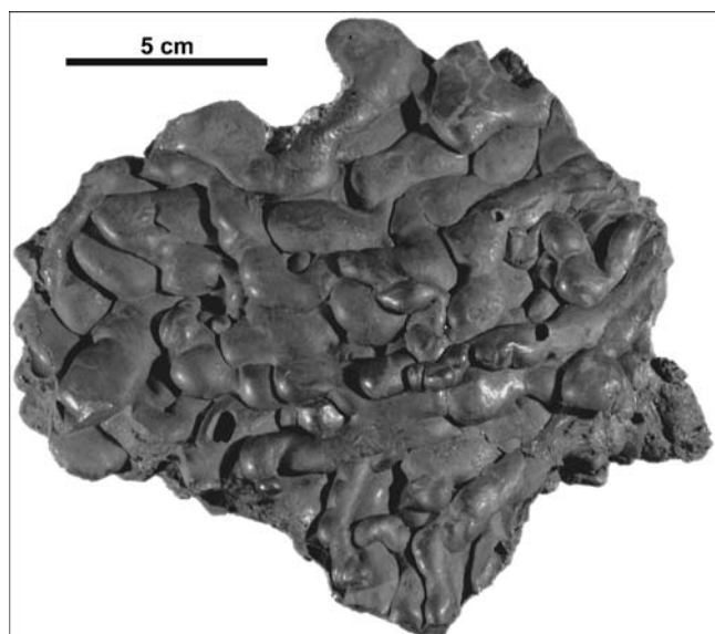
Abb. 8. Fließschlacke aus der Schlackenhalde bei der Ulrichsbrücke. Die wurmförmigen Fließstränge, die nur bei sehr dünnflüssigen Schmelzen entstehen, sind charakteristisch für diesen auffälligsten und häufigsten Schlackentyp der Füssener Gegend. Fließschlacken entstehen beim „Schlackenabstich“, bei dem die flüssige Schlacke während oder am Ende des Ofenbetriebes abgelassen wird (vgl. Abb. 2). Probe U7732.
