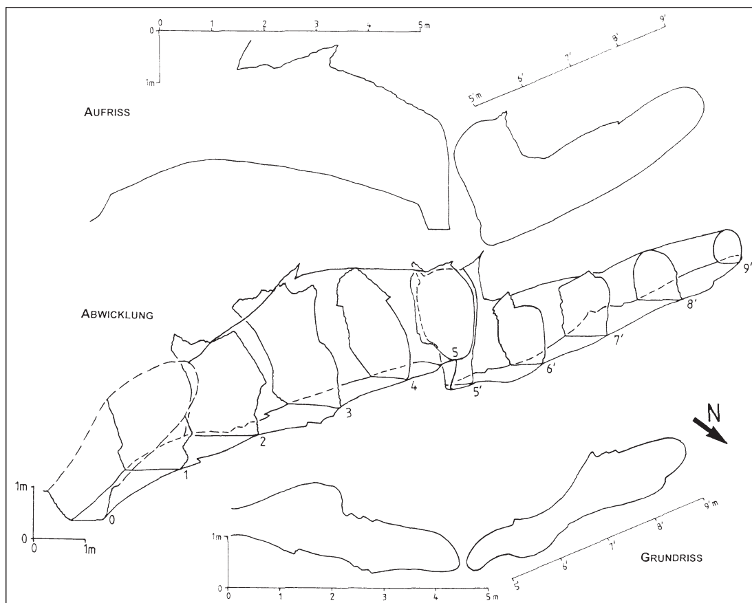
Abb. 20. Grundriss, Abwicklung und Aufriss der Karsthöhle bei Unterpinswang, die als potentieller Abbaustollen diskutiert wird. Bei der Abwicklung sind die Querschnitte maßstäblich, der Verlauf der Sohle und der Firste verzerrt.
