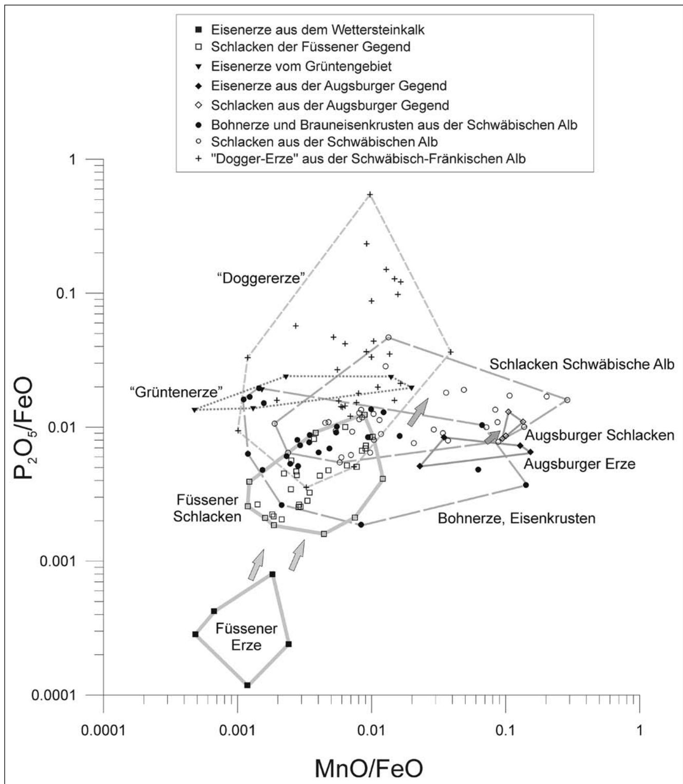
Abb. 5. \text{MnO}/\text{FeO} - \text{P}_2\text{O}_5/\text{FeO} -Verhältnisse der Erze aus dem Oberen Wettersteinkalk und der Schlacken aus der Füssener Gegend sowie verschiedener Eisenerze (und Schlacken) aus der näheren und weiteren Umgebung (vgl. Abb. 4). Die Pfeile deuten auf die Anreicherung der Elemente im Rennfeuerprozess hin. Die Umgrenzungen der einzelnen Felder dienen ausschließlich der besseren Lesbarkeit der Abbildung und haben keine analytische oder statistische Bedeutung. Datengrundlage: Tab. 3, BÖHNE (1963), FEHR (2000), FISCHER & HAUNER (1987), FRANK et al. (1975), FREI (1966), FRÖHLICH (1984), MUTSCHLECHNER (1955), SCHNEIDERHÖHN (1980), TAUPITZ (1954 a), YALÇIN & HAUPTMANN (1995).
