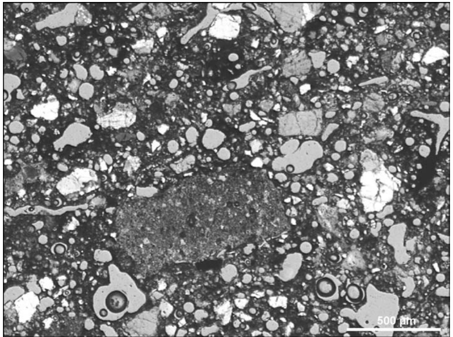
Abb. 13. Dünnschliffbild einer glasig-porösen Probe. In einer glasigen Matrix (dunkel) sind zahlreiche Quarzbruchstücke (weiß-grau) eingelagert, die nicht aufgeschmolzene Reste der Ofenwand darstellen. Die Probe enthält unzählige, meist runde Blasen Hohlräume (hellgrau). Durchlicht; Polarisatoren zu ca. 45° gekreuzt. Lokalität Roßhaupten, Probe OR7725.
