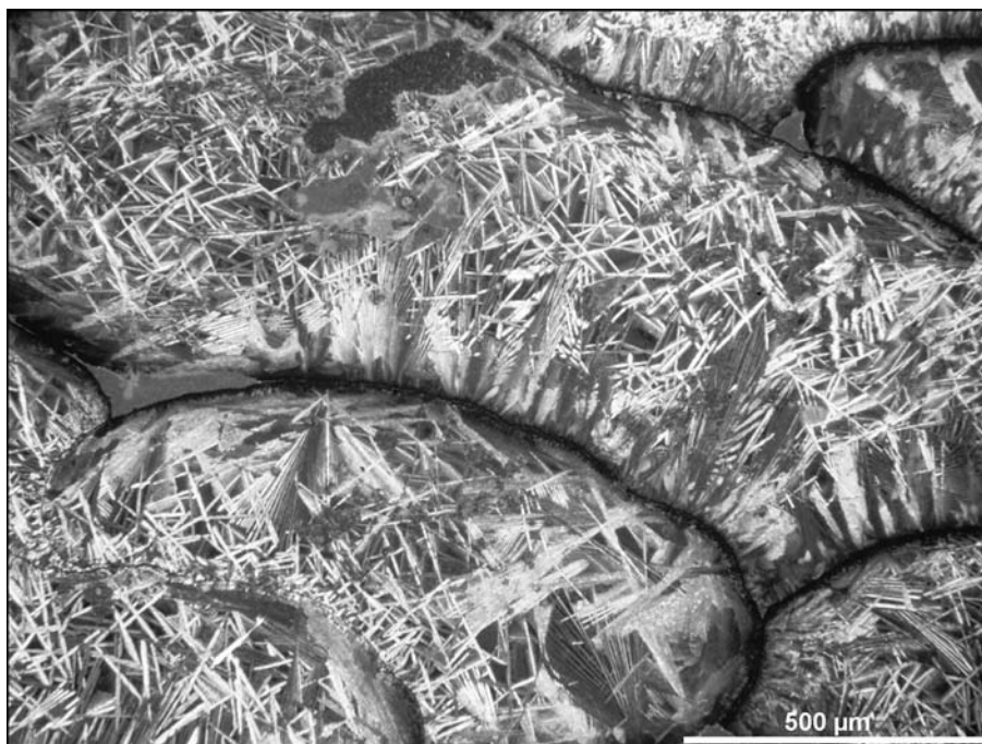
Abb. 11. Dünnschliffbild einer fayalitischen Fließschlacke.
