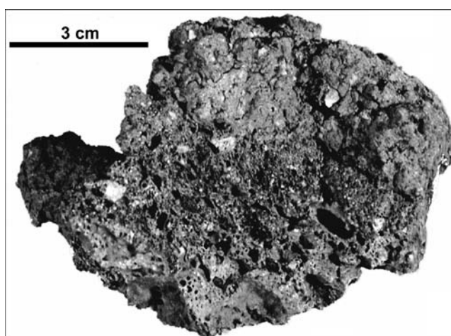
Abb. 10. Glasig-poröses Material aus der Schlackenhalde bei Osterreinen. Im unteren Bereich ist eine glasige Masse mit unzähligen, meist runden Poren sowie einigen hellen Quarz- und Gesteinsbruchstücken zu erkennen. Der obere Bereich ist weniger porös, zeigt Risse und ist randlich sehr brüchig. Das glasig-poröse Material ist keine Schlacke, sondern ein Reaktionsprodukt zwischen der Schmelze und der sandig-lehmigen Ofenwand. Probe OR7726.
