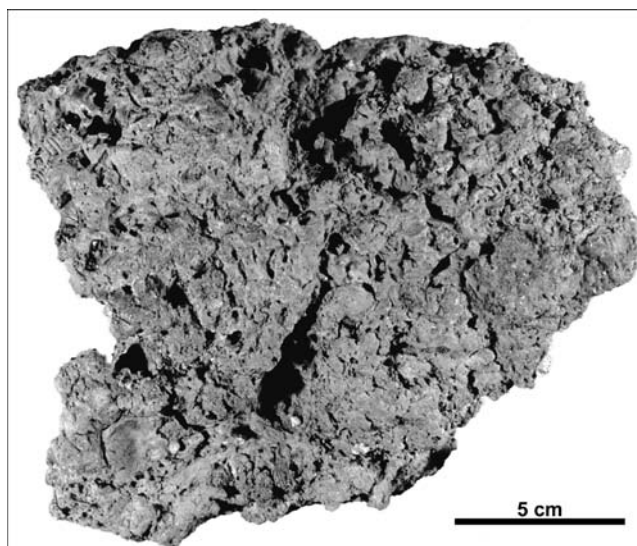
Abb. 9. Heterogene Schlacke aus der Schlackenhalde bei der Ulrichsbrücke. Die rostigen Verwitterungsfarben sind eine Folge der zahlreichen metallischen Eiseneinschlüsse. Neben Eiseneinschlüssen kennzeichnen diesen Schlackentyp das Fehlen von Fließstrukturen, die unregelmäßig zellig-kavernöse Struktur und eingeschlossene Holzkohlestückchen. Die Holzkohlereste weisen darauf hin, dass die heterogenen Schlacken innerhalb des Ofens entstanden sind (vgl. Abb. 2). Probe U7743.
