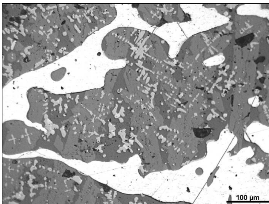
Abb. 12. Anschliffbild einer heterogenen, metallreichen Schlacke.
