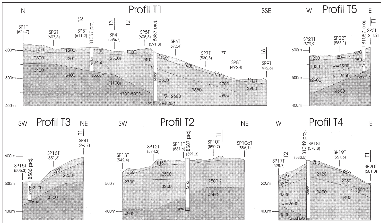
Abb. 3. Refraktionsseismische Profile T1–T5.
