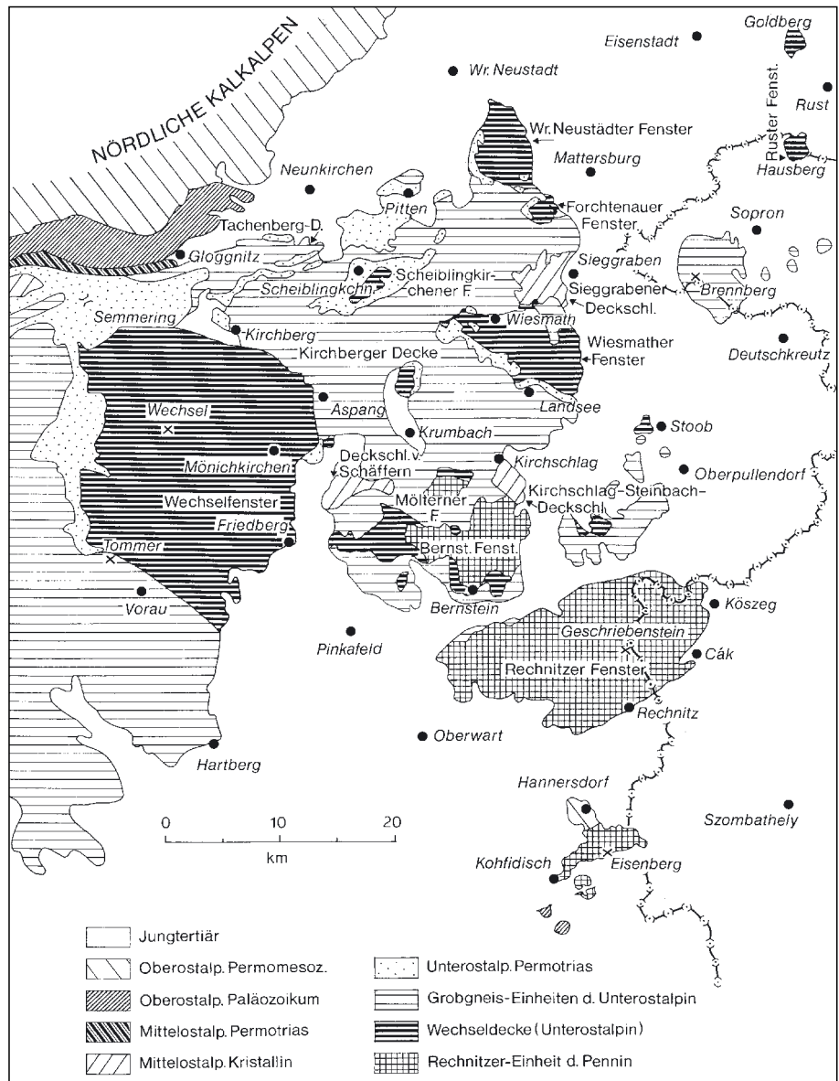
Abb. 1. Geologische Übersicht des Nordostsporns der Zentralalpen. Aus P. HERRMANN & A. PAHR (1988) nach A. TOLLMANN (1978).
