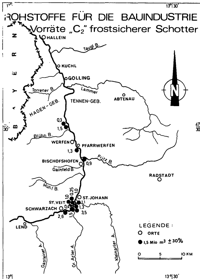
Abb. 9: Vorräte „C2“ frostsicherer Schotter im Salzachtal zwischen Golling und Schwarzach.
