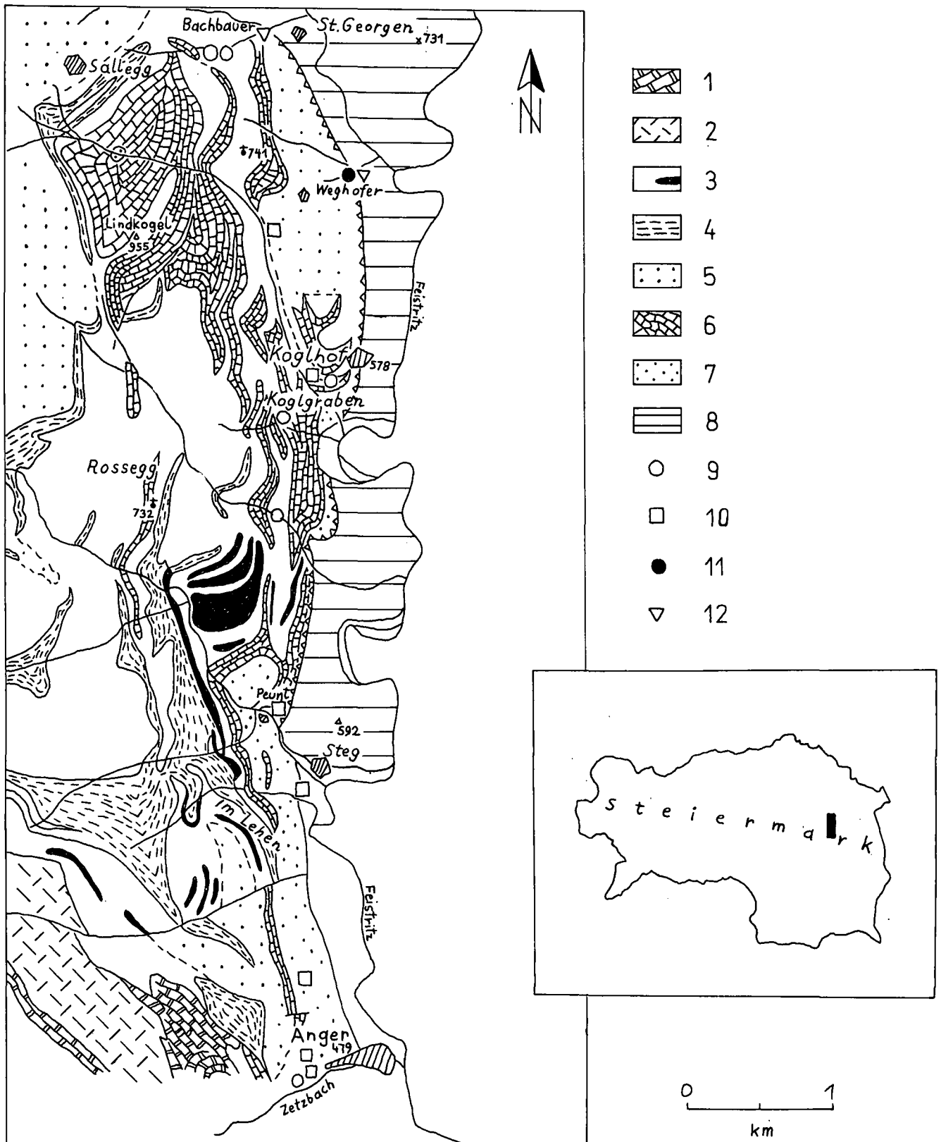
Abb.1: Die Vorkommen von Pegmatiten (einschließlich besonderer Rollstücke) im Angerkristallin, eingetragen in die geologische Karte von F. NEUBAUER 1981, Abb. 1 (verändert).
