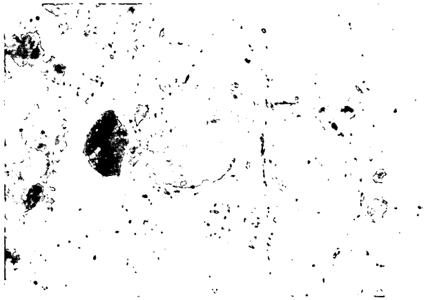
Abb. 2: Stark verschiefelter Pegmatit mit großen Spodumenblasten und feinkörnigem Spodumenpflaster (entlang der Schieferungsflächen) in einer feinkörnigen Quarz-Feldspat-Matrix. E Weghofer (Abb. 1), Nicols ||, Bildbreite ca. 20 mm.
