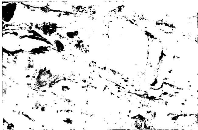
Abb. 7: Große Spodumenblöcke mit feinkörnigem Spodumen (Bruchstück!) und Granat (dunkle Fahnen) entlang der Schieferungsflächen. Vorkommen wie in Abb. 3; Nicols ||, Bildbreite ca. 20 mm.
