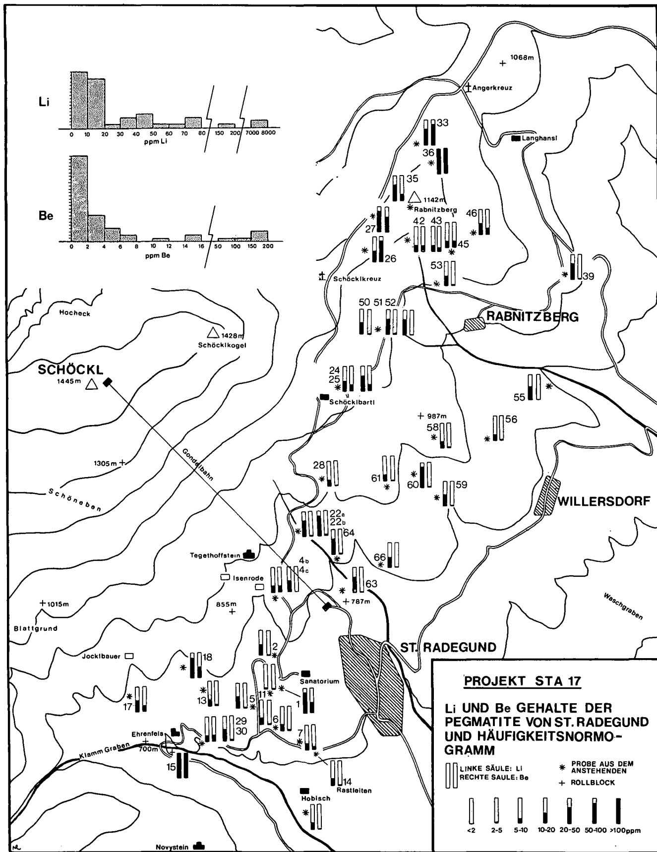
Abb. 8: Lithium- und Beryllium-Gehalte der Pegmatitproben von St. Radegund und Umgebung mit Häufigkeitsnormogramm. Die aufgetragene Strecke der Gondelbahn entspricht 2000 m.
