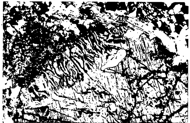
Abb. 4: Myrmekitische Verwachsung von Spodumen und Albit am Rande eines großen Spodumenkristalles. Randlich treten zerscherzte, feinkörnige Spodumenaggregate in einer Quarz-Albit-Matrix auf; Vorkommen wie Abb. 3; Nicols x, Bildbreite ca. 1,8 mm.
