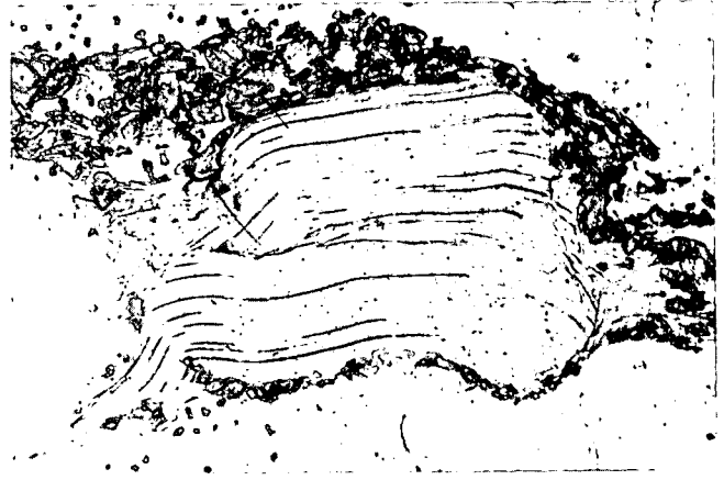
Abb. 3: Stark deformierter Muskovitkristall von feinkörnigem, phengitischem Hellglimmer, Spodumen und Granat umgeben. Das umgebende Quarz-Feldspatgefüge ist rekristallisiert. Probe Ra 36, N-Hang Rabnitzberg, St. Radegund, Nicols ||, Bildbreite ca. 1,8 mm.
