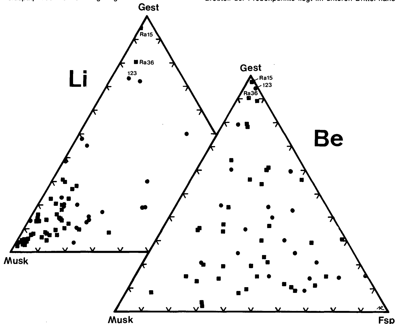
Abb. 13: Dreiecksdarstellung der Analysendaten von den Pegmatiten und ihren Muskovit- und Feldspatkonzentrationen für Lithium und Beryllium. Symbole siehe Abb. 10.
