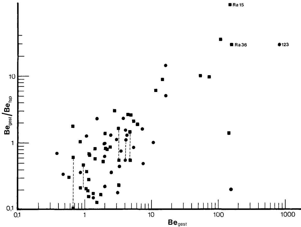
Abb. 11: Korrelationsdiagramme Be_{Gest} gegen Be_{Gest}/Be_{Musk} und Be_{Gest}/Be_{Fsp} . Symbole siehe Abb. 10.
