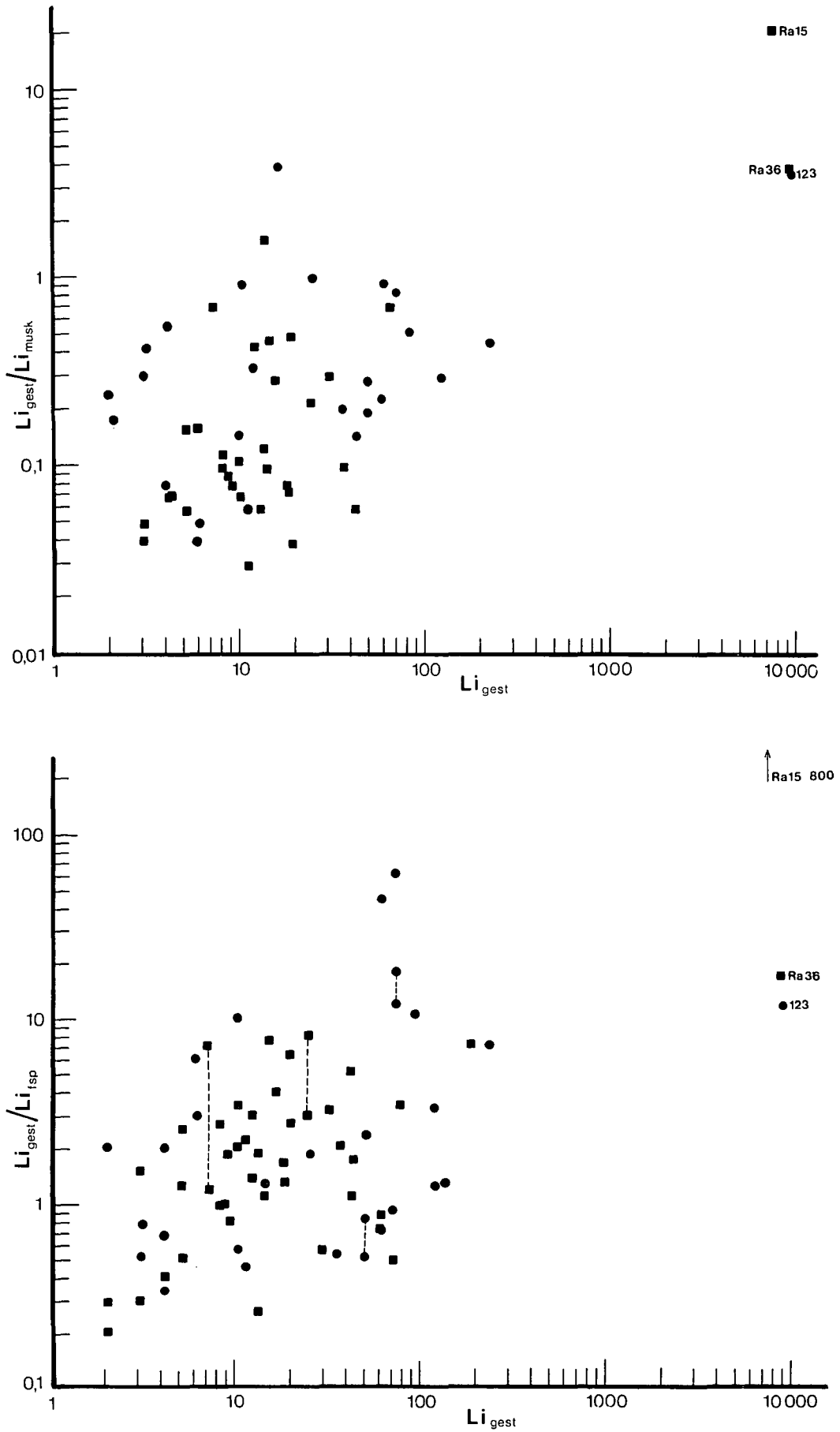
Abb. 10: Korrelationsdiagramme Li_{gest} gegen Li_{gest}/Li_{Musk} und Li_{gest}/Li_{Fsp} . Mit ■ wurden die Proben aus dem Kristallin von St. Radegund eingetragen, mit ● die der Gleinalpe. Die Projektionspaare koexistierender Feldspatpaare wurden miteinander verbunden, die Spodumenpegmatitpunkte wurden beschriftet (Ra 15, Ra 36 und 123), Konzentrationsangaben in ppm.
