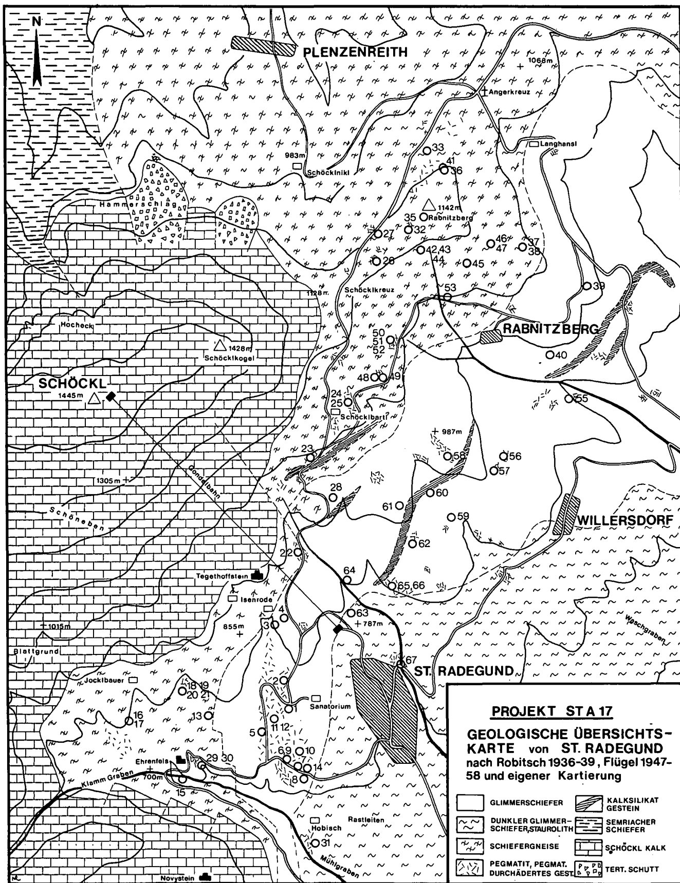
Abb. 1: Geologische Übersichtskarte von St. Radegund und Umgebung (nach ROBITSCH, 1949; FLÜGEL, 1960 und eigener Kartierung) mit eingetragenen Probenpunkten (Ra 1 – Ra 67). Die aufgetragene Strecke der Gondelbahn entspricht 2000 m.
