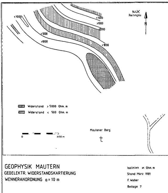
Abb. 7: Geoelektrische Widerstandskartierung.
