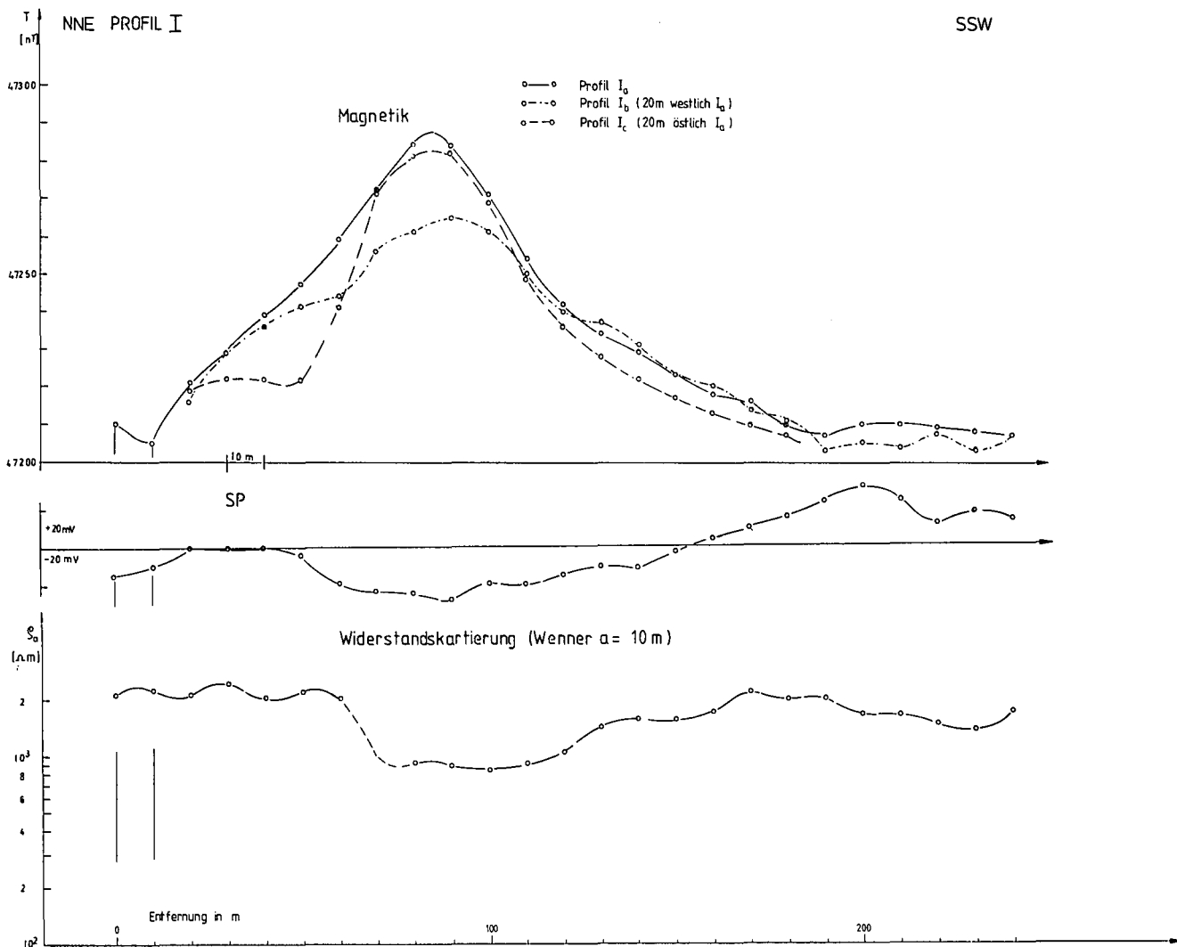
Abb. 9: Geophysik Kammern – Profil I (Magnetik, SP, Widerstandskartierung); Stand Dezember 1980.
