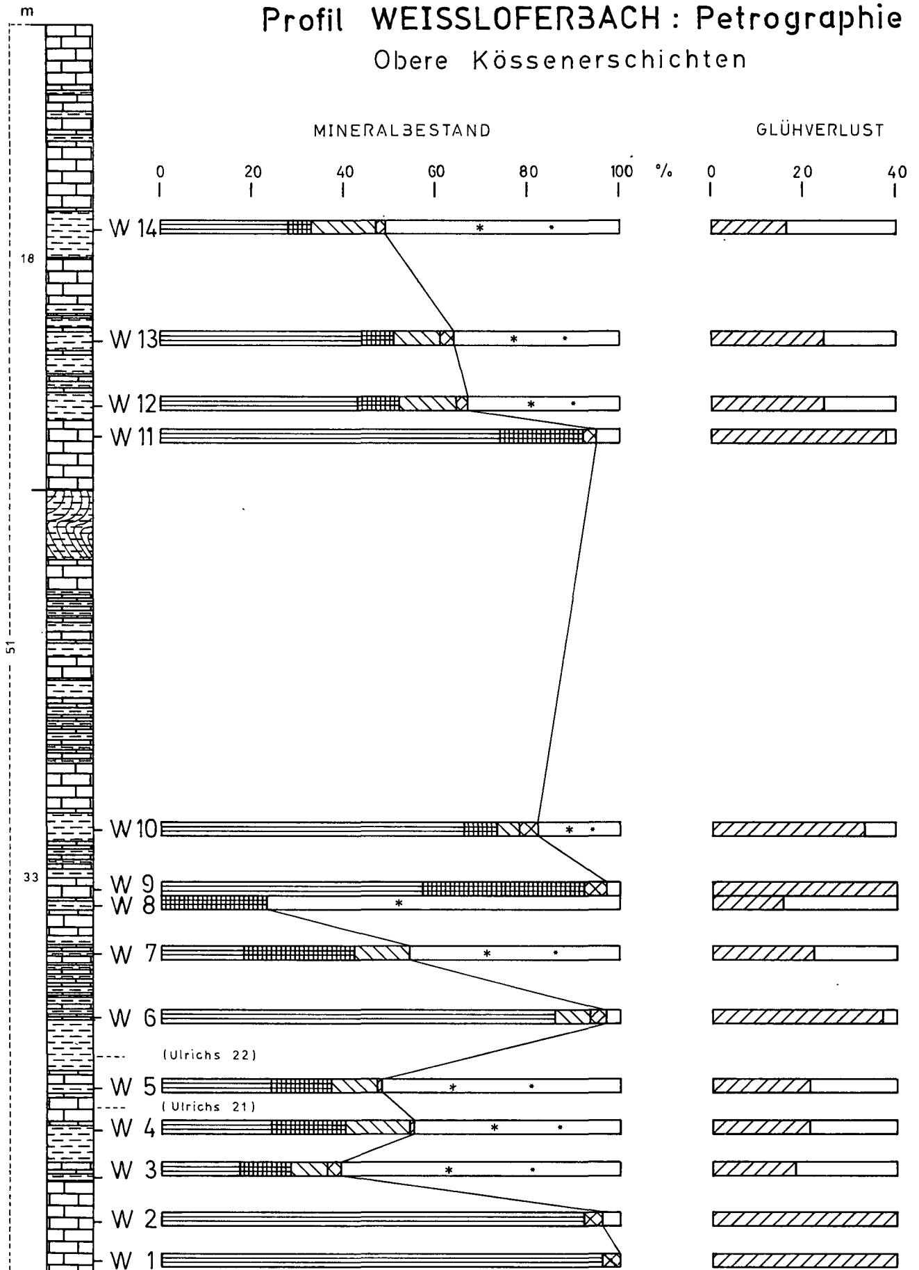
Abb. 5: Profil und Mineralbestand; Vorkommen Weißloferbach, Kössener Schichten.
