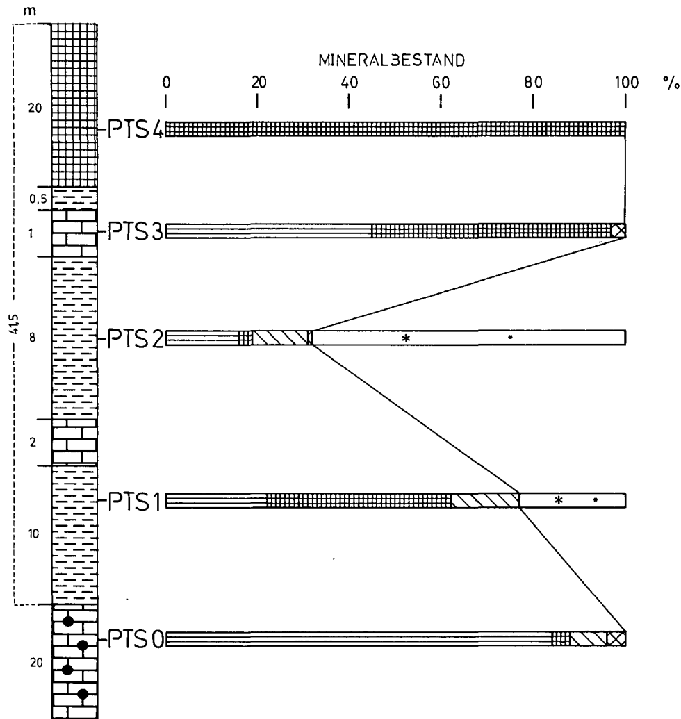
Abb. 3: Profil und Mineralbestand; Vorkommen Thaur, Partnach-Schichten.
