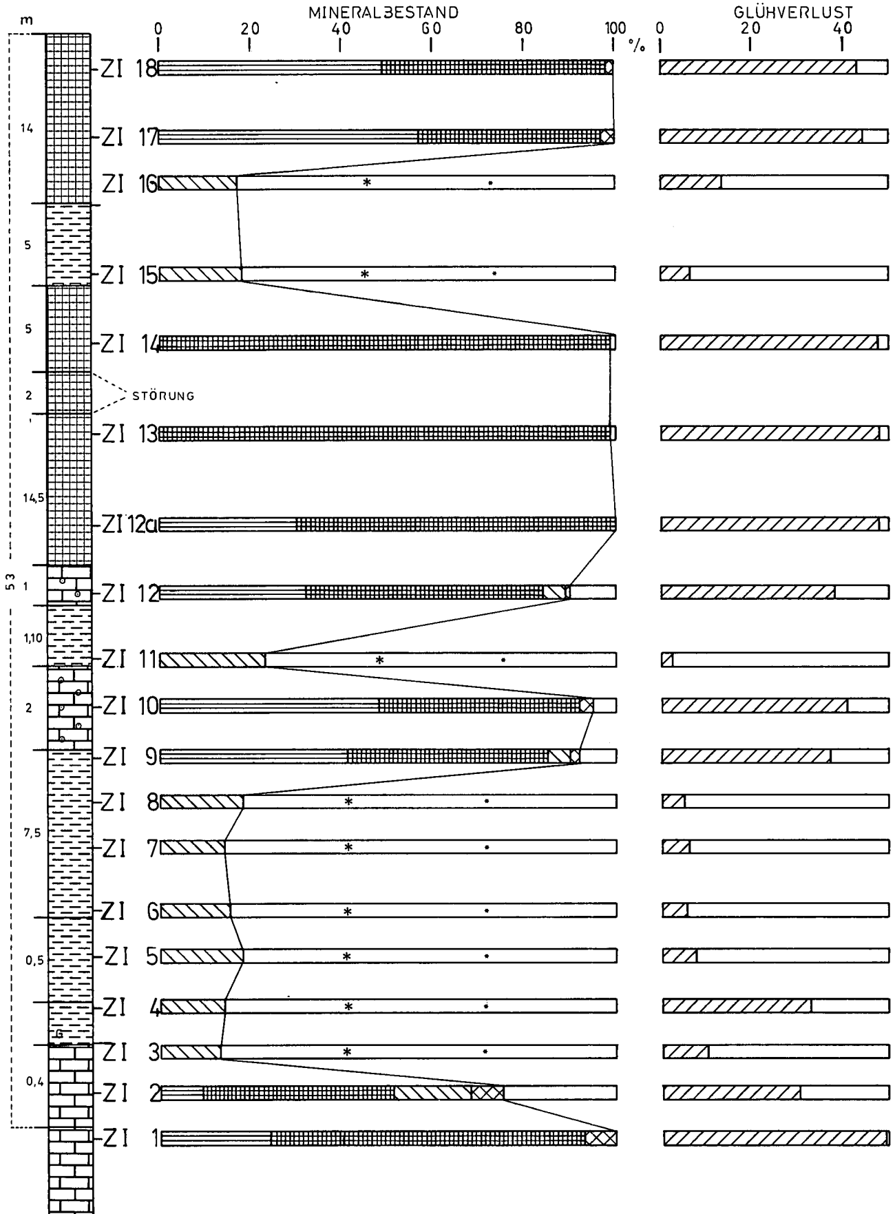
Abb. 4: Profil und Mineralbestand; Vorkommen Zirl, Raibler Schichten, tiefster Schieferhorizont am Kalvarienberg.
