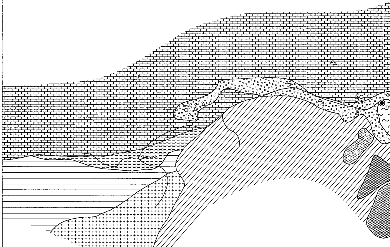
Abb. 1: Übersichtsskizze der Geologie von Tirol mit Probelokalitäten zur Tonanalyse.
