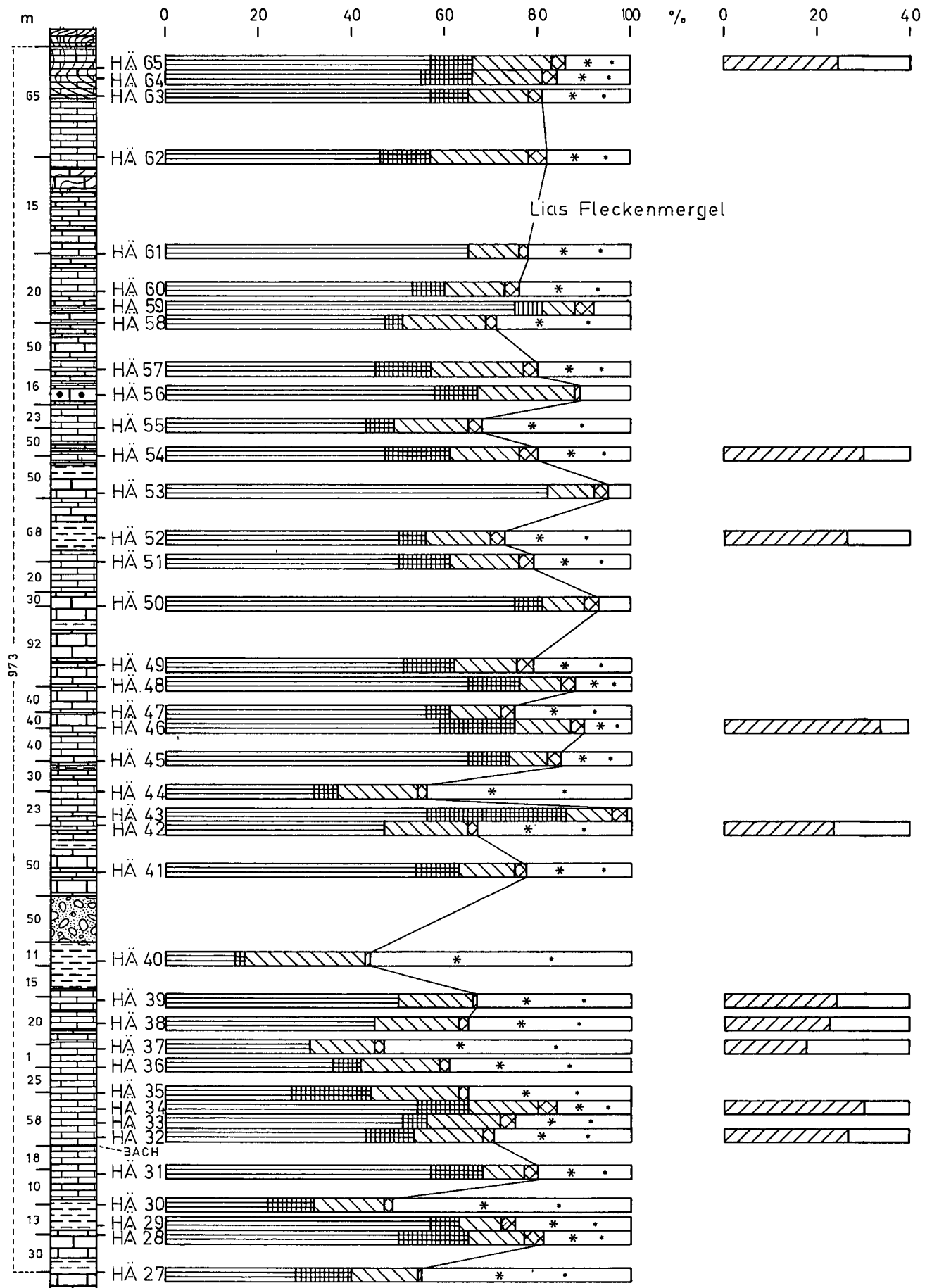
Abb. 6: Profil und Mineralbestand; Vorkommen Häselgehr, Allgäuschichten.
